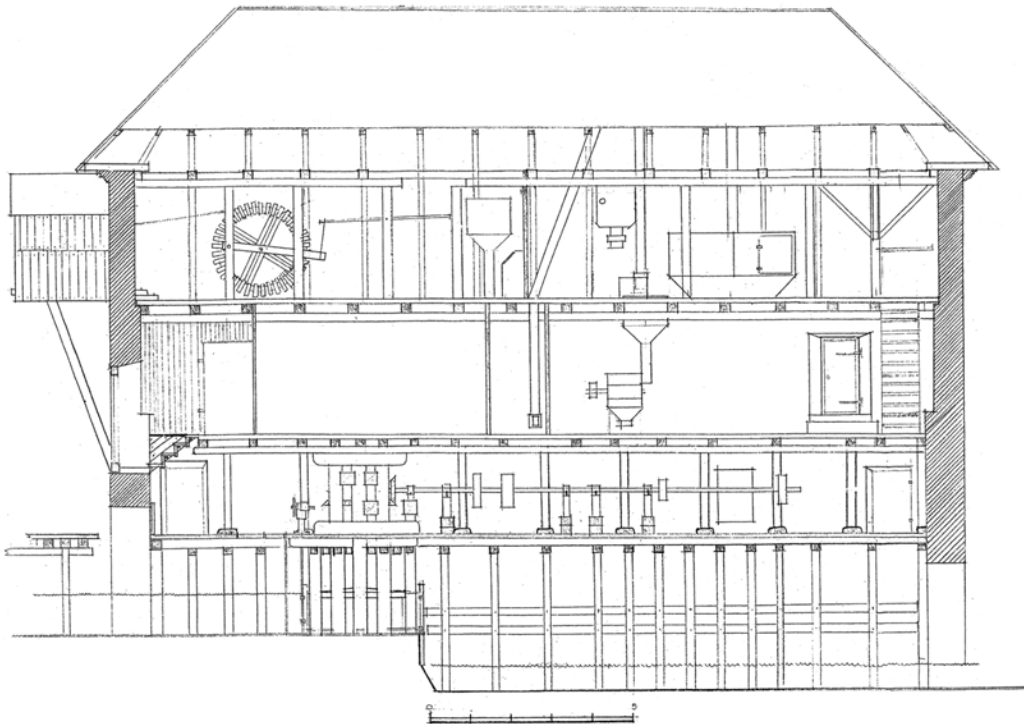
8 pav. Dvaro malūno pjūvis. KTU ASIA
