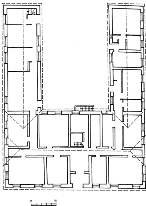
3 pav. Dvaro administratoriaus namo planas.
