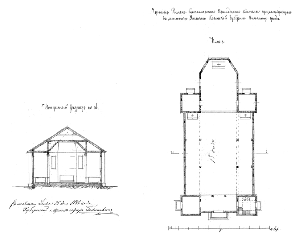
11 pav. Medinės Užpalių bažnyčios apmatauimo brėžiniai (planas ir pjūvis). KAA, f. I-473, ap. 2, b. 11, l. 1
