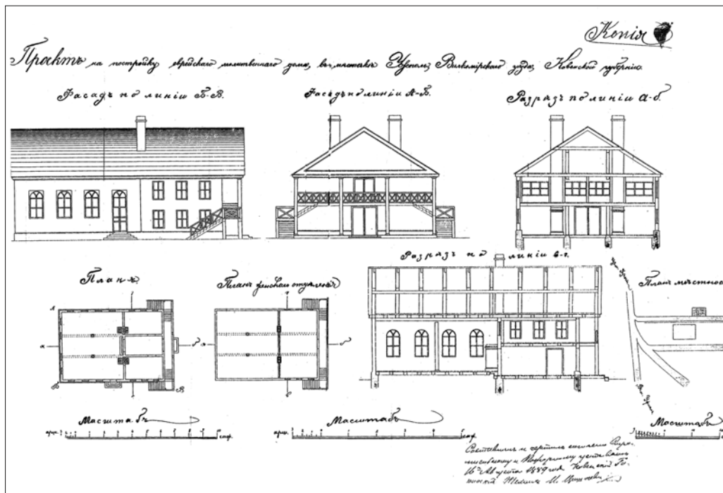
14 pav. Užpalių sinagogos projektas. KAA, f. I-49, ap. 1, b. 15840, l. 3334
