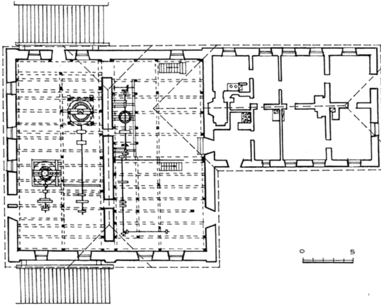
7 pav. Dvaro malūno planas. KTU ASIA
