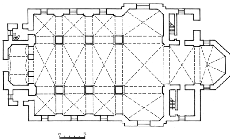
12 pav. Bažnyčios plano schema. 2010 m. Sudarė A. Rupeika
