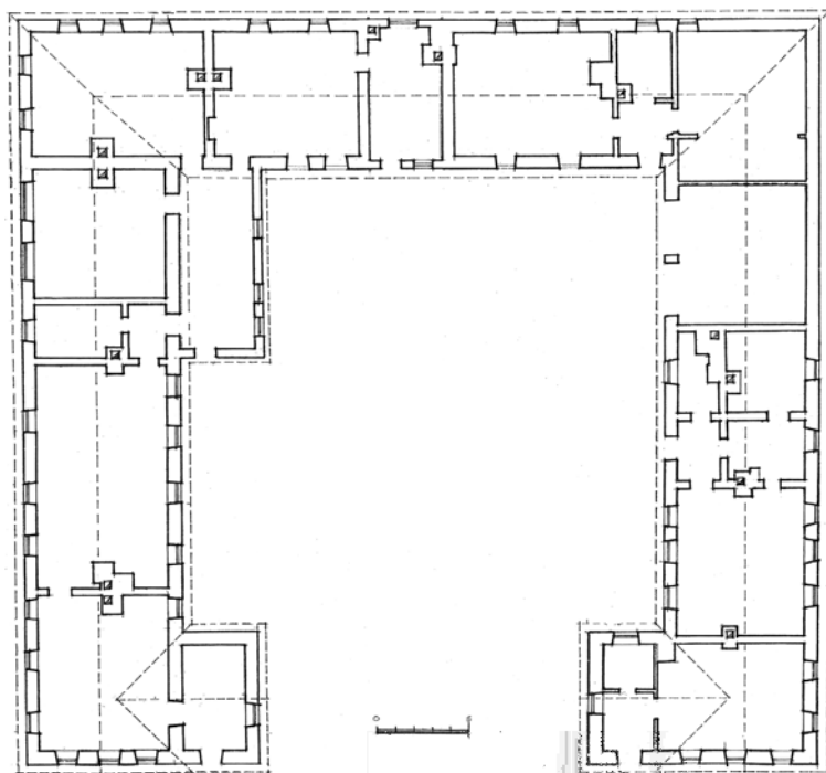
5 pav. Dvaro tvarto planas. KTU ASIA
