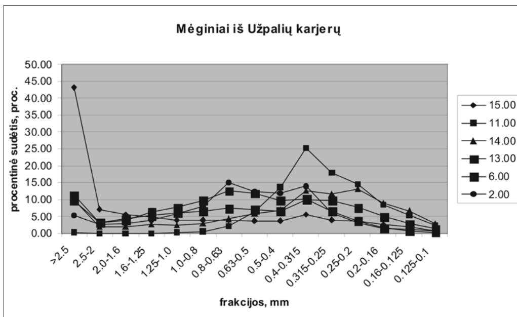
4 pav. Karjerų nuogulų granulimetrinės sudėties grafikas. Sutartiniai ženklai atitinka 1 lentelę
