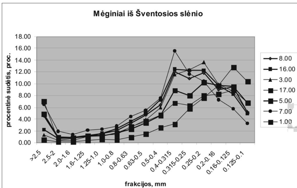
5 pav. Šventosios slėnio nuogulų granulimetrinės sudėties grafikas. Sutartiniai ženklai atitinka 1 lentelę. (Žr. splv. 2, 3 pav. Šeimyniškių atodanga ir konglomerato uola)
