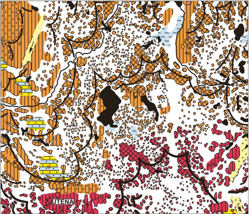
1 pav. Užpalių apylinkių geomorfologinis žemėlapis. Pagal Č. Kudabą, 1983 m.
