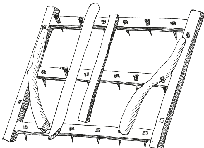
5 pav. Rėminės akėčios. VU BRS, f. 81, b. 255
