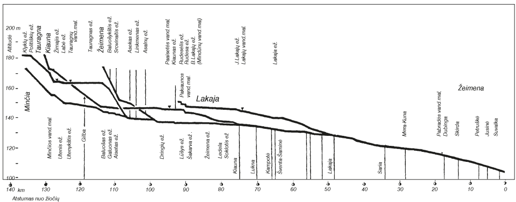
26 pav. Išilginiai Tauragnos, Minčios, Kiaunos, Lakajos ir Žeimenos upių profiliai
