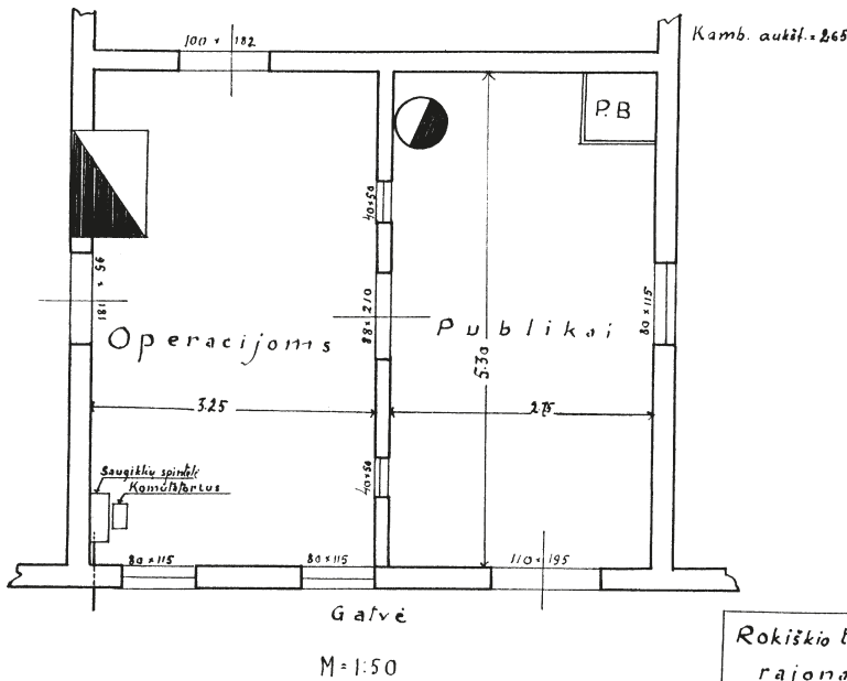
Tauragnų pašto įstaigos planas. 1936 m. LCVA, f. 1016, ap. 2, b. 175, l. 3
