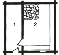
6 pav. Pirties planas:
