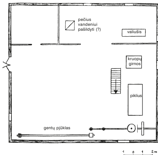
7 pav. Minčios vėlyklos pirmojo aukšto planas
