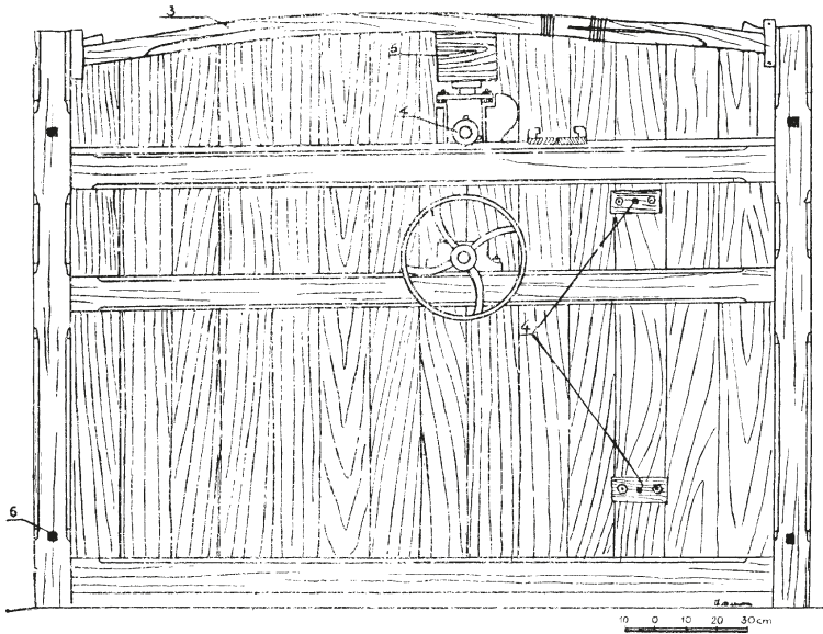
5 pav. 1 – pagrindinis velenas, 2 – judamojo veleno ašis, 3 – lingė, 4 – išlyginamųjų velenų guoliai, 5 – paveržimo kaladėlės, 6 – rėmo sutvirtinimo varžtai
