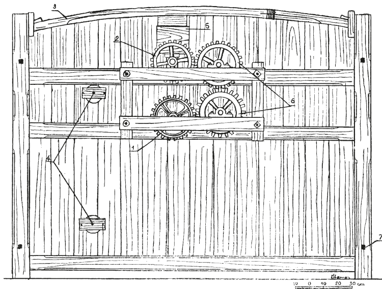
6 pav. 1 – pagrindinio veleno dantratis, 2 – judamojo veleno dantratis, 3 – lingė, 4 – išlyginamųjų velenų guoliai, 5 – paveržimo kaladėlė, 6 – perdavimo dantračiai, 7 – rėmo sutvirtinimo varžtai
