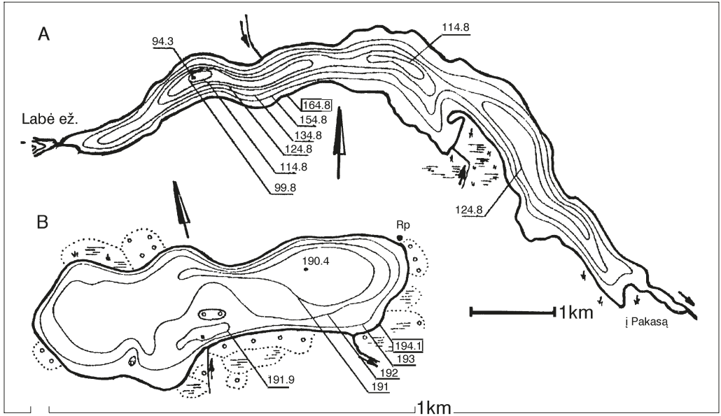
25 pav. Dvejopų rininių ežerų dubenų palyginimas: A – giluminė atsikūrusi Tauragno ežero rina ir B – paviršiuje silpnai išreikšta atsikūrusi Vaikeso ežero rina
