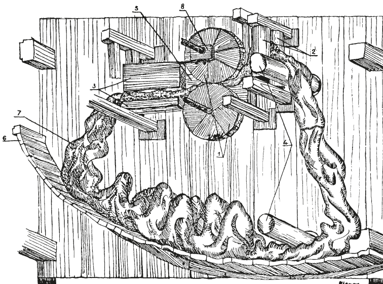
2 pav. 1 – vėlimo velenai, 2 – nukreipimo velenai, 3 – kūlokai, 4 – išlyginamieji velenai, 5 – vėlimo velenų ir kūlokų dėžė, 6 – valiušo grindys, 7 – milas, 8 – viršutinis kūloko guolis
