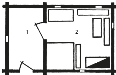
1 pav. Seniausias aukštaitiškas sodybos trobesys – dūminė pirkia. 1 – priemenė, 2 – pirkia.
