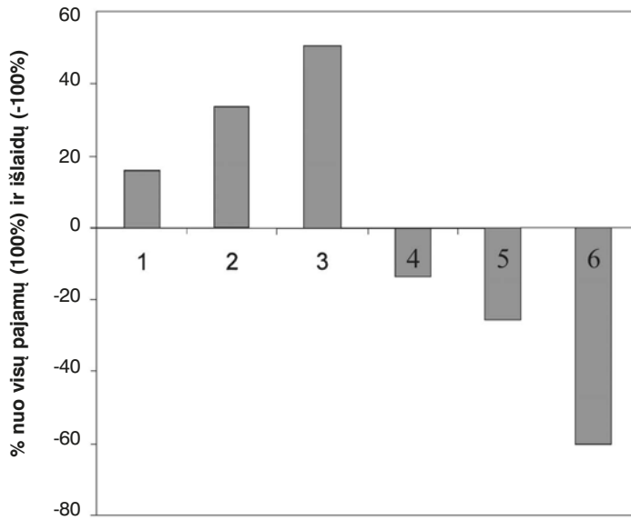
3 pav. Tauragno ežero vandens balanso (vidutinio daugiamečio) struktūra. Vandens pajamos: 1 – krituliai, išskrintantys ant ežero paviršiaus, 2 – paviršinė prietaka upeliais ir ežero šlaitais, 3 – požeminė prietaka. Vandens išlaidos: 4 – garavimas iš ežero vandens paviršiaus, 5 – nuotėkis Tauragnos upeliu, 6 – filtracija (požeminis nuotėkis)
