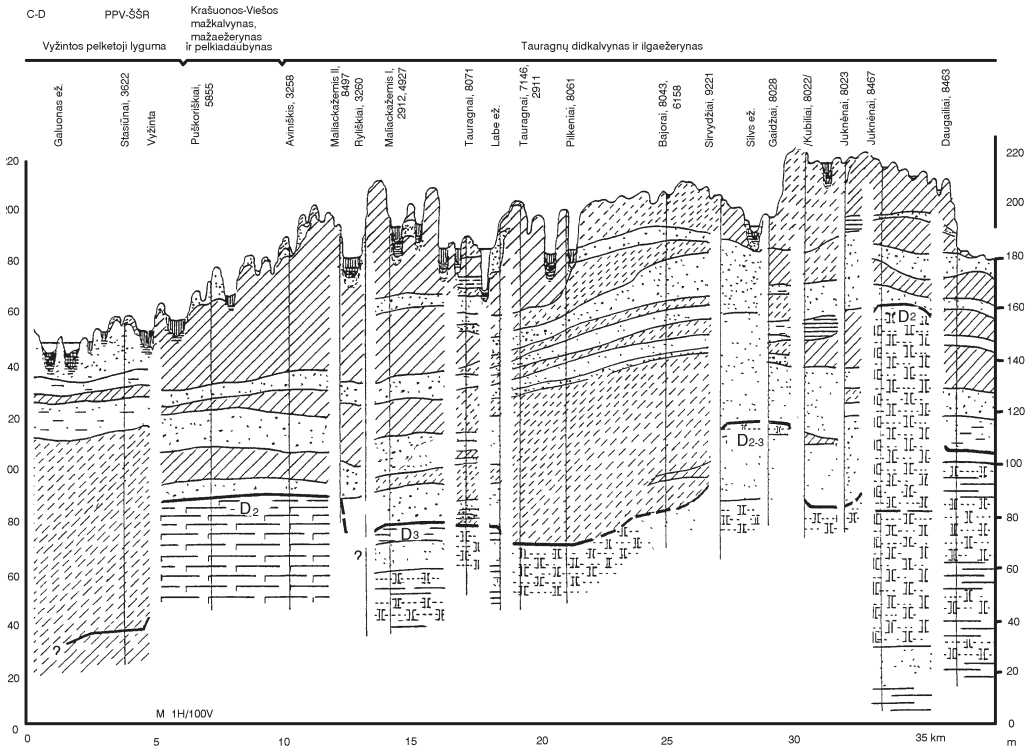
5 pav. Vyžintos pelkėtosios lygumos ir Tauragnų didkalvyno geologinis profilis (sudarė R. Kunskas)
