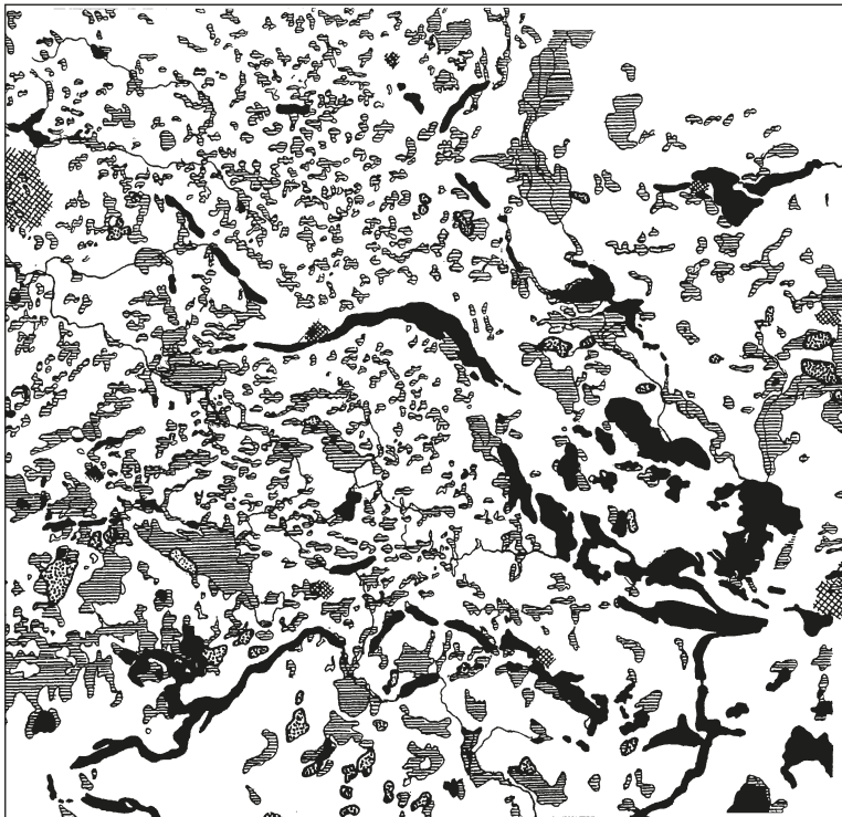
28 pav. Skirtingas pelkynų tankumas ir pelkių forma įvairiose aukštumų ir lygumų vietovėse (sudarė R. Kunkskas)
