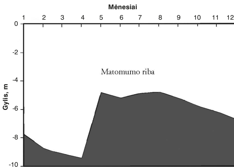
2 pav. Vandens skaidrumo (balto skritulio matomumo ribos) kaita Tauragno ežere (1963 m. duomenys)
