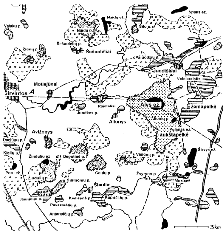
Rytinio širvintų lygumos pakraščio Širvintos ir Musės aukštumų pelkynas
