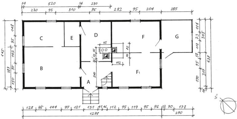
10 pav. Gyvenamojo namo, statyto 1934 m., planas. Kirmiškių k. Braižė D. Sabaliauskienė
