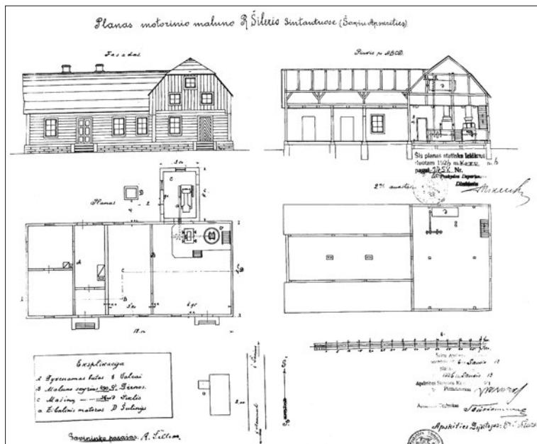
68 pav. R. Šilerio motorinio malūno planas
