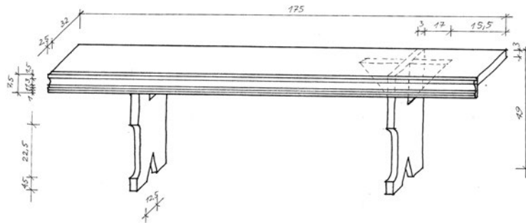
29 pav. Suolas. 1929 m. Kirmiškių k. Braižė D. Sabaliauskienė
