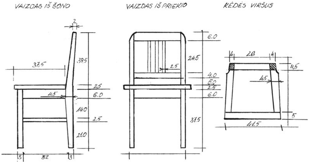
35 pav. Kėdė. 1930 m. Sintautų mstl. Braižė Jurgita Paškevičiūtė
