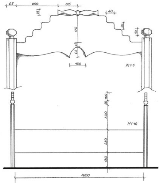
37 pav. Lova. 1907 m. Urbantų k. Braižė I. Mikštaitė
