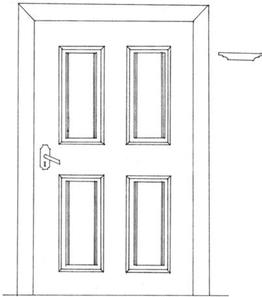
19 pav. Gyvenamojo namo, statyto XIX a. pab., durys iš priebučio į stubą. Gaisrių k. Braižė A. Miliauskaitė
