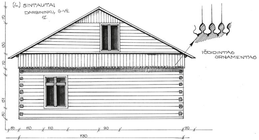
12 pav. Gyvenamojo namo fasadas. Sintautų k. Braižė Gaila Stulgaitytė
