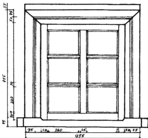
2 pav. Šesiarūtis langas (mm)
