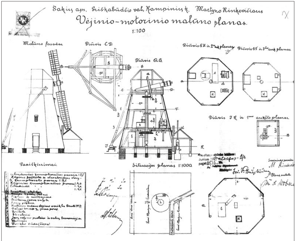
64 pav. M. Rinkevičiaus vėjo-motorinio malūno planas
