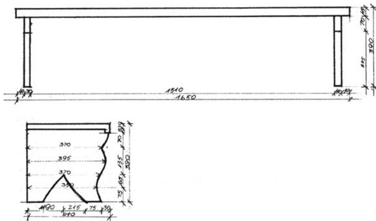
30 pav. Suolas. Sintautų mstl. Braižė V. Mostauskytė
