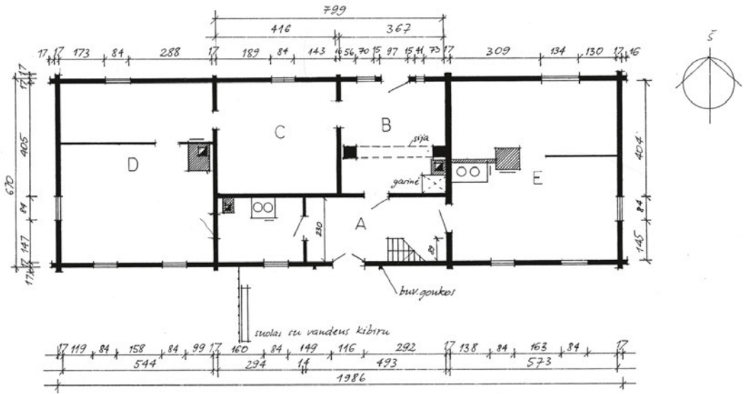
4 pav. Gyvenamojo namo, statyto apie 1900 m., planas. Voverių k. Braižė D. Sabaliauskienė
