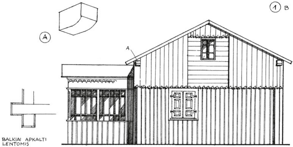
8 pav. Gyvenamojo namo, statyto 1923 m., fasadas iš pietų pusės. Bliūkiškių k. Braižė D. Šulgaitė
