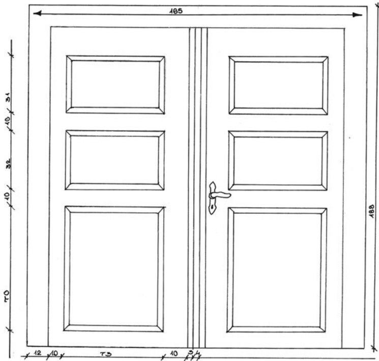
22 pav. Gyvenamojo namo doivėrės vidaus durys įstiklintu viršumi. Sintautų mstl. Braižė G. Stulgaitytė
