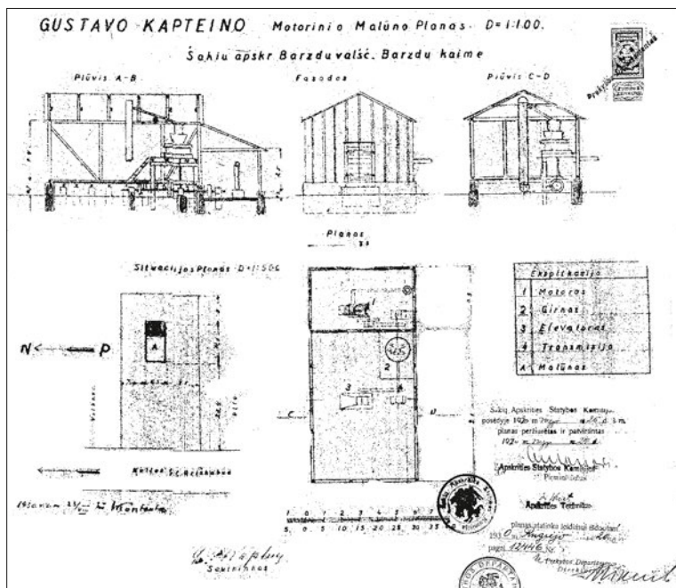
38 pav. Gustavo Kapteino motorinio malūno Barzdų k. planas
