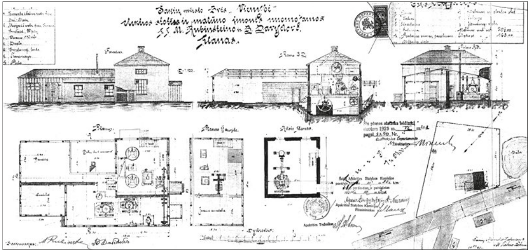
50 pav. Šakių miesto bendrovės „Vienybė“ Šakių elektros stoties ir malūno įmonės planas
