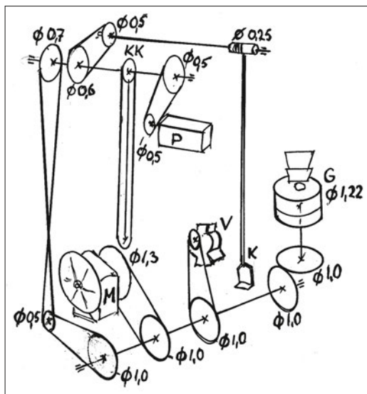
67 pav. K. Skinkio malūno kinematinė schema
