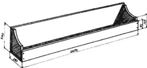
3 pav. Lentyna virš stubos durų (mm)
