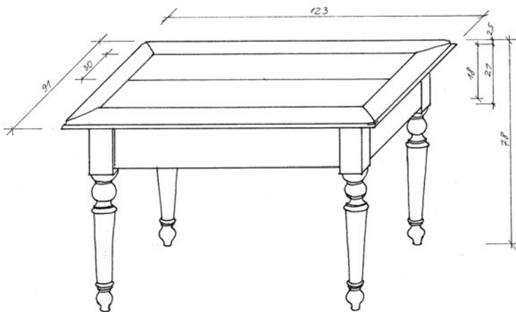
25 pav. Stalas. XIX a. pr. Kirmiškių k. Braižė D. Sabaliauskienė
