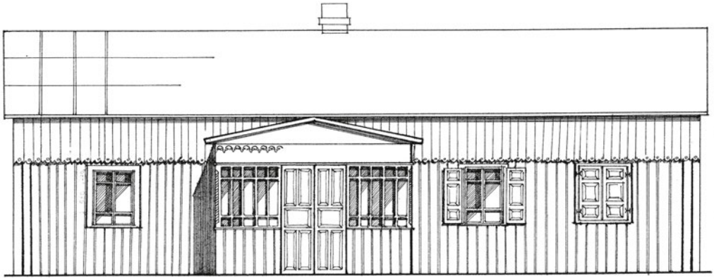
VAKARINIS FASADAS M 1:50
