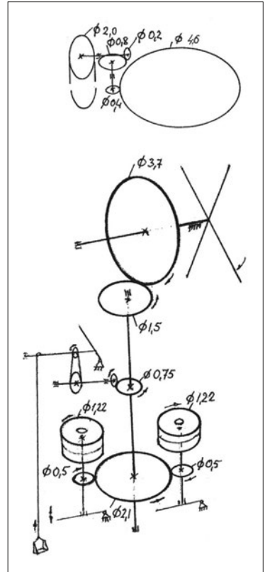
46 pav. Antano Rinkevičiaus vėjo malūno Birštonų k. kinematinės schemos
