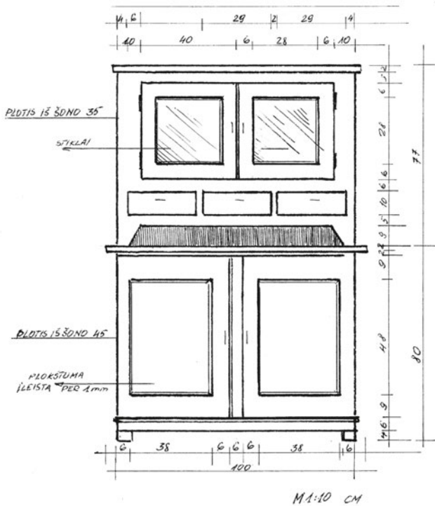
48 pav. Indų spinta. XX a. pr. Sintautų mstl. Braižė L. Bomblauskienė
