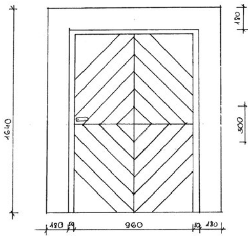
VAIZDAS IŠ PRIEKIO M 1:20
