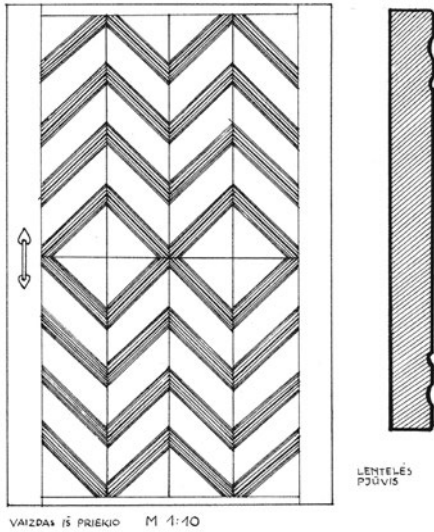
15 pav. Gyvenamojo namo, statyto XIX a., durys. Keturnaujienos k. Braižė D. Šulgaitė
