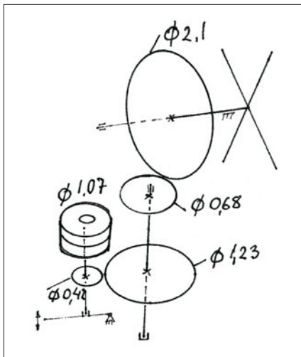
18 pav. Dvapakopė girnų sukimo pavara
