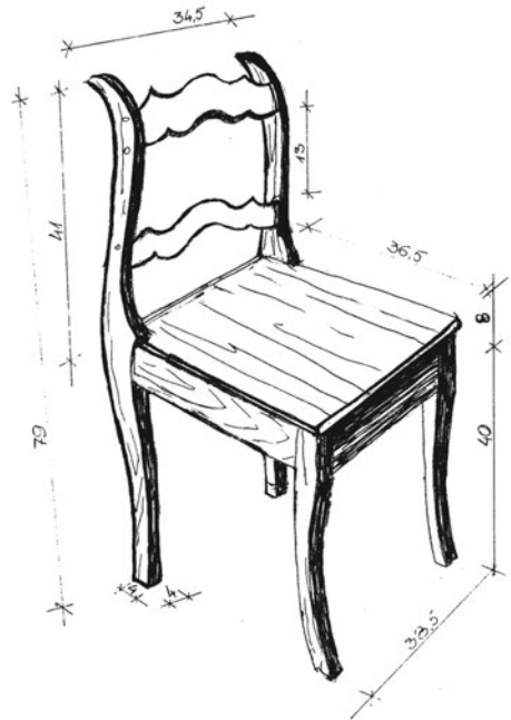
34 pav. Kėdė. XIX a. pab. Braižė
