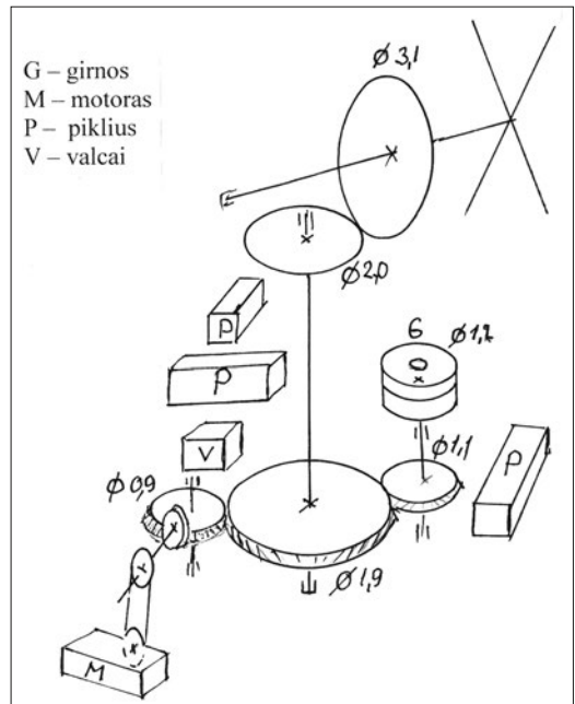
61 pav. A. Ešiaus malūno kinematinė schema
