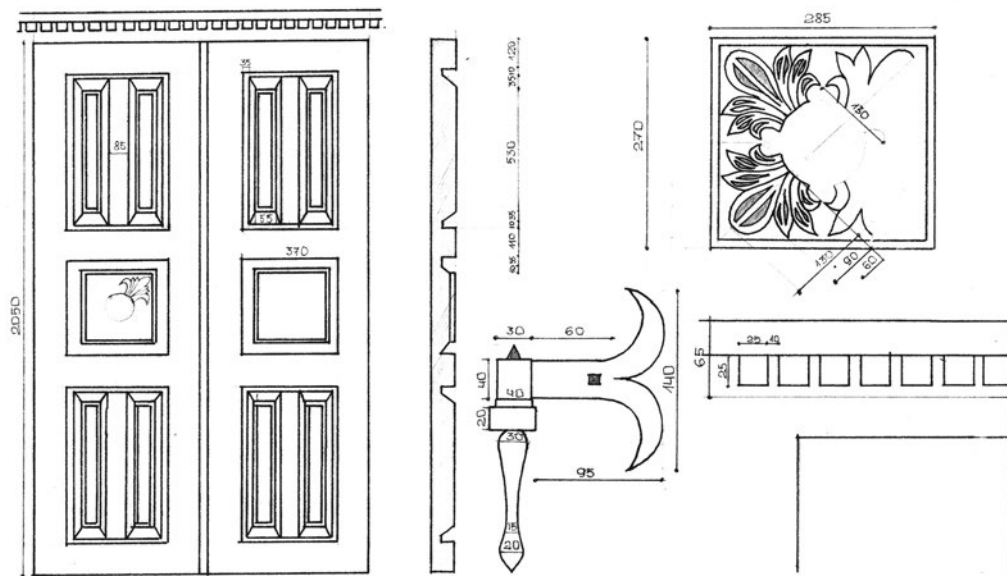
17 pav. Gyvenamojo namo, statyto 1923 m., dvišerės durys su išprūdomis. Bliūkiškių k. Braižė Visata Gaputytė
