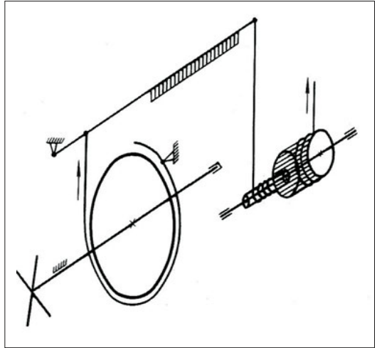
15 pav. Stabdžio kinematinė schema
