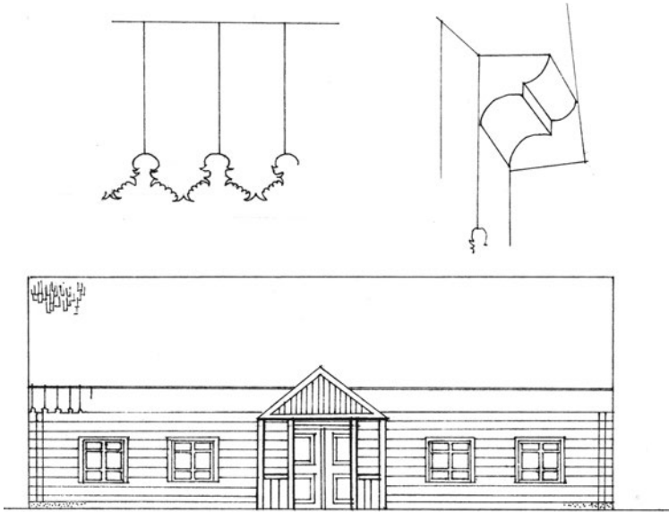
5 pav. Gyvenamojo namo, statyto 1917 m., rytinis fasadas. Gaisrių k. Braižė Auksė Miliauskaitė
