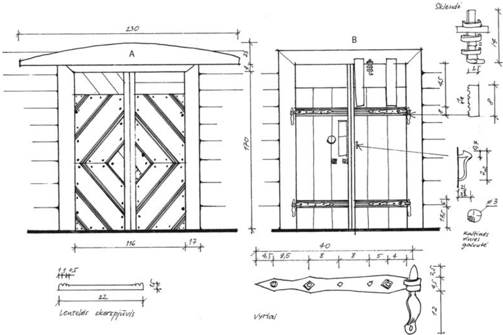
16 pav. Gyvenamojo namo dviverės durys. Voverių k. Braižė D. Sabaliauskienė
