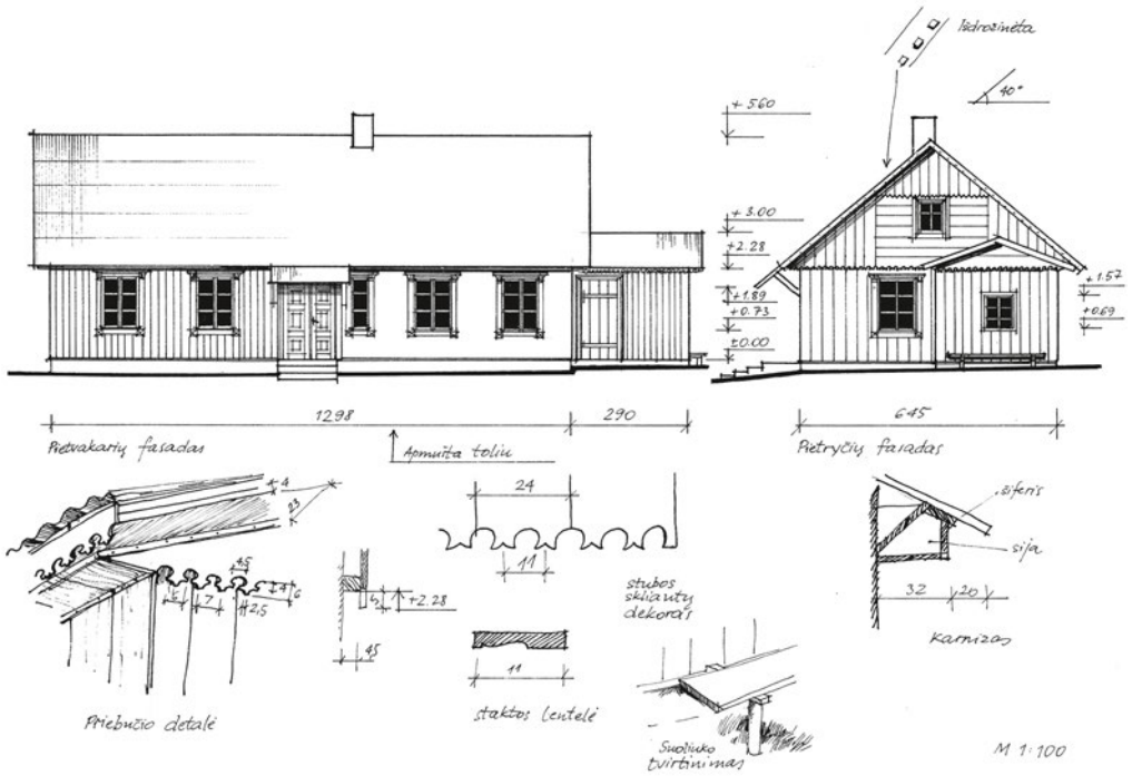
9 pav. Gyvenamojo namo, statyto 1934 m., fasadai ir jų detalės. Kirmiškių k. Braižė D. Sabaliauskienė
