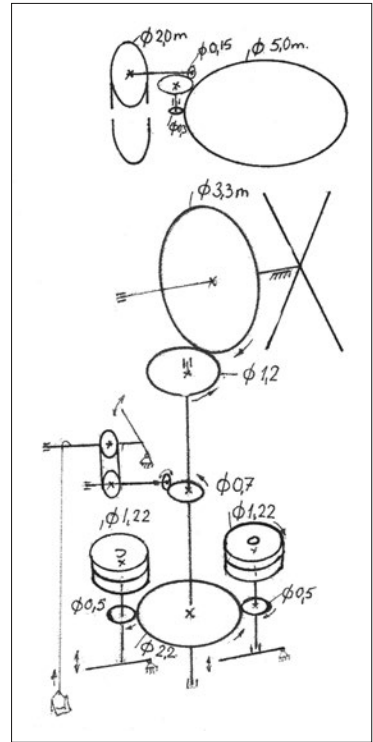
30 pav. Prano Kuro Kiaulupių k. kepurinio vėjo malūno kinematinės schemos
