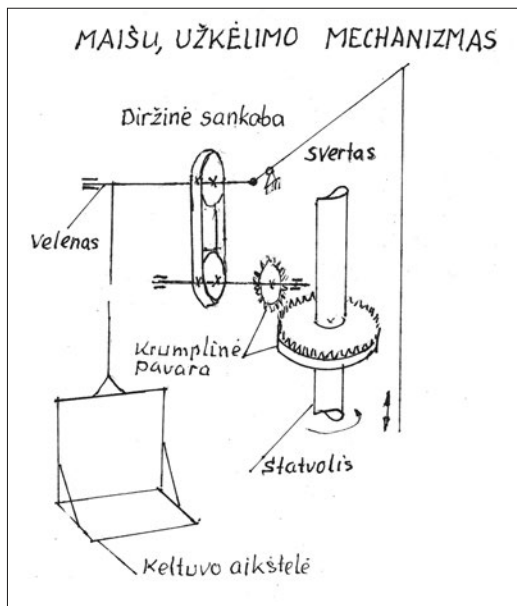
13 pav. Maišų užkėlimo mechanizmo kinematinė schema
