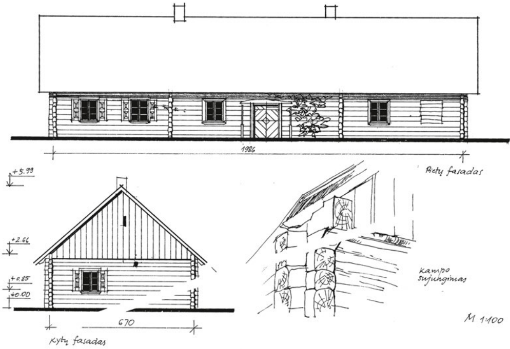
2 pav. Gyvenamojo namo, statyto apie 1900 m., fasadas. Voverių k. Braižė D. Sabaliauskienė
