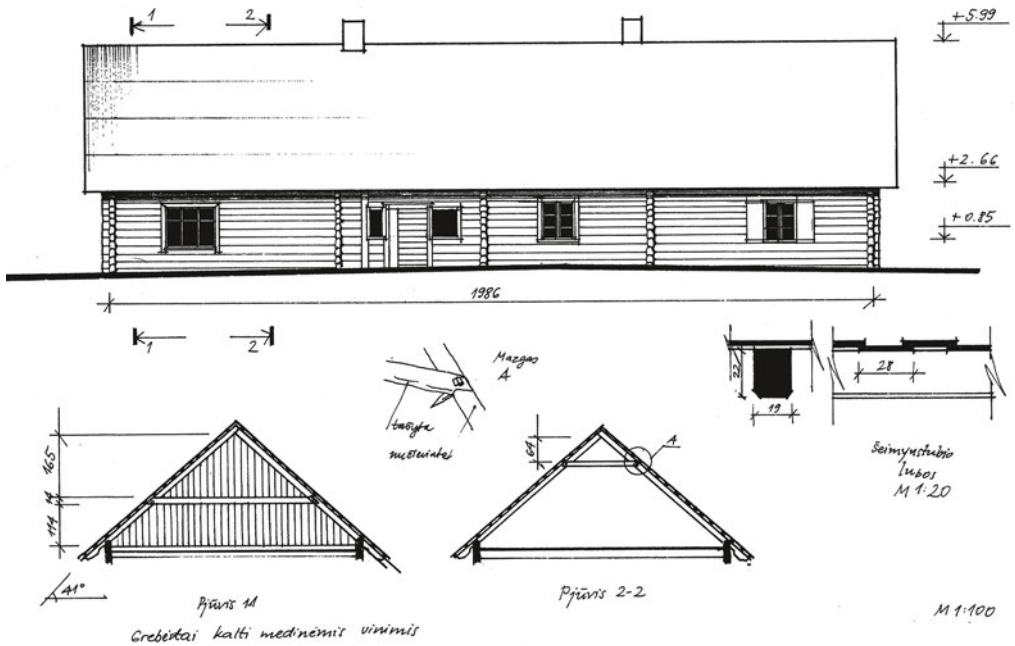
3 pav. Gyvenamojo namo, statyto apie 1930 m., fasadas, pjūvis, fragmentai. Voverių k. Braižė D. Sabaliauskienė
