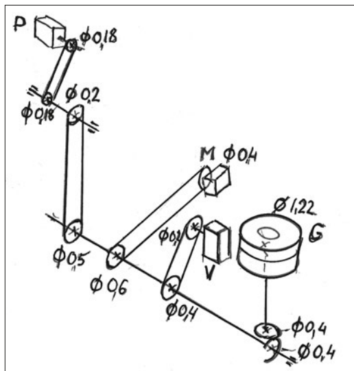
69 pav. R. Šilerio motorinio malūno kinematinė schema
