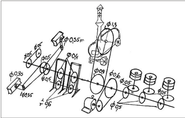
56 pav. Oskaro Vingendorfo malūno ir lentpjūvės transmisijos schema
