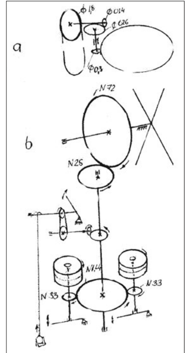
26 pav. Rygiškių malūno kinematinės schemos: a) kepurės apgręžimo krumpliaratine pavara kinematinė schema, b) malūno ir maišų užkėlimo mechanizmo kinematinė schema
