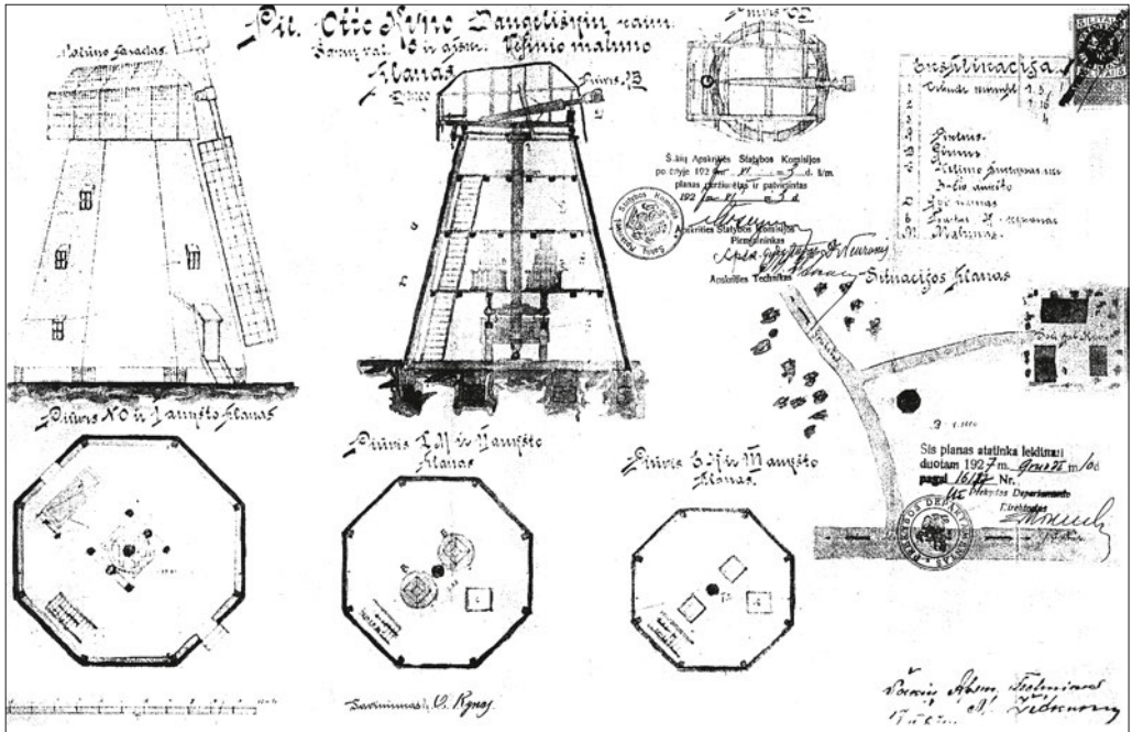
39 pav. Otto Kyno vėjo malūno Daugėliškio k. planas
