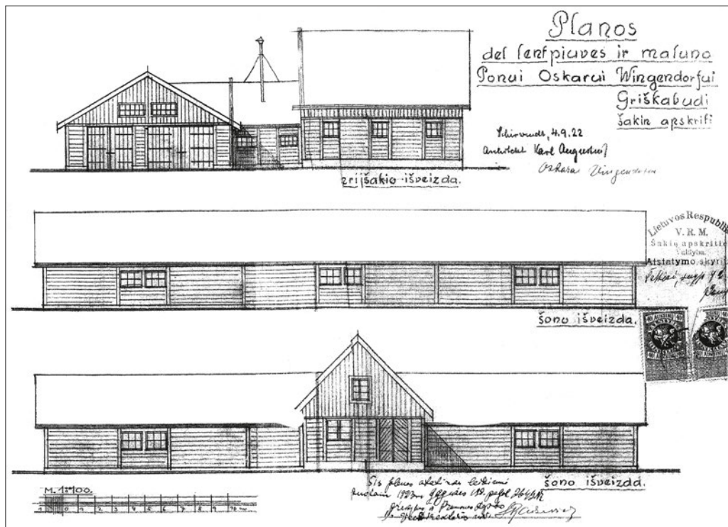
54 pav. Oskaro Vingendorfo lentpjūvės ir malūno fasadai
