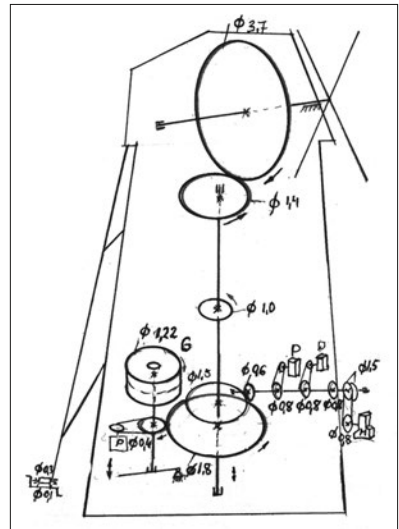
65 pav. M. Rinkevičiaus malūno kinematinė schema
