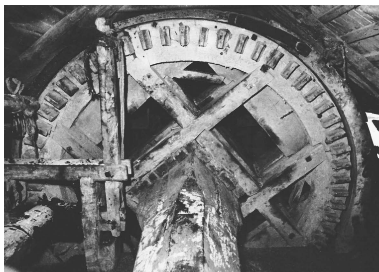
14 pav. Juostinis medinis malūno stabdys
