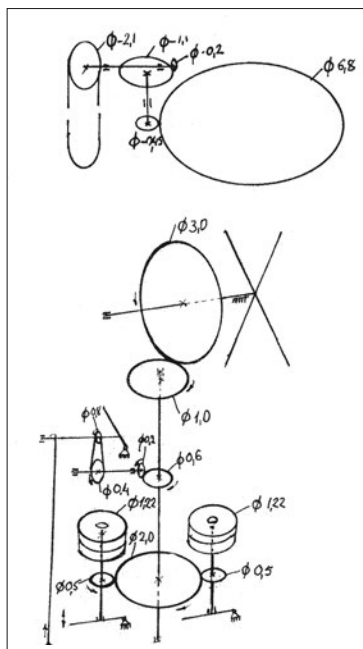
33 pav. Augusto Cakryzos kepurinio vėjo malūno Pranskabūdžio k. kinematinės schemas
