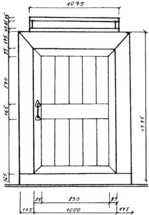
4 pav. Durys iš stubos į priemenę (mm)
