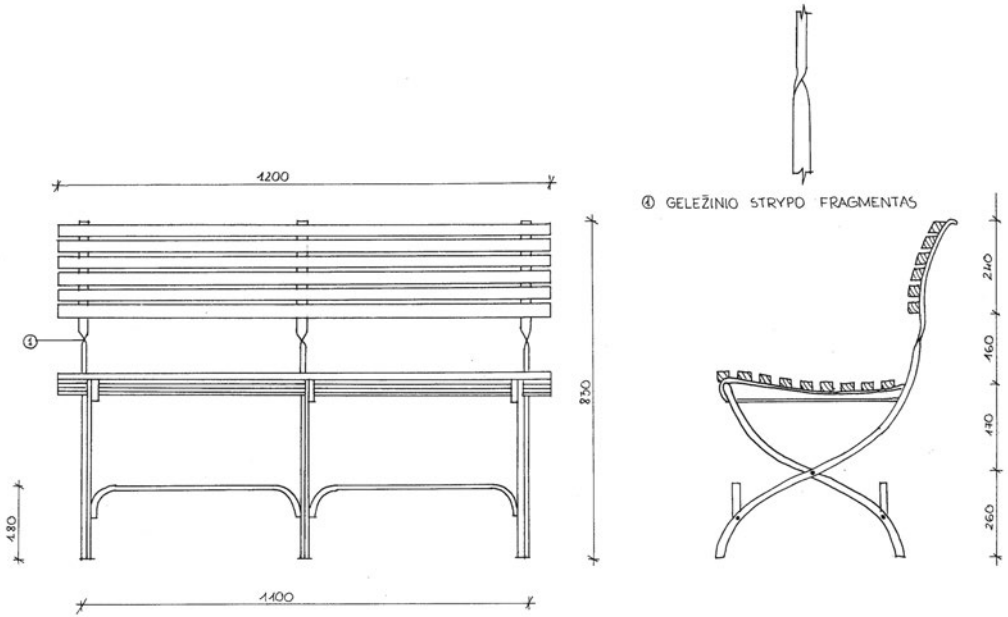
31 pav. Suolelis. Sintautų mstl. Braižė S. Stadalninkaitė
