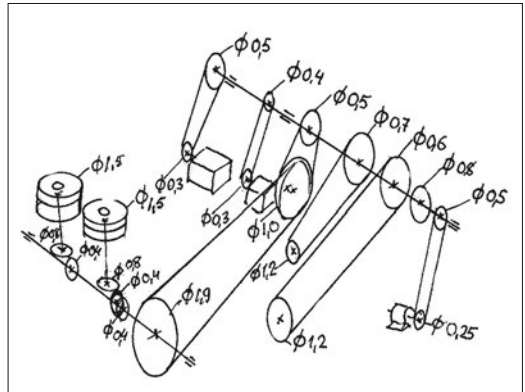
51 pav. Šakių miesto bendrovės „Vienybė“ Šakių elektros stoties ir malūno įmonės transmisijos schema
