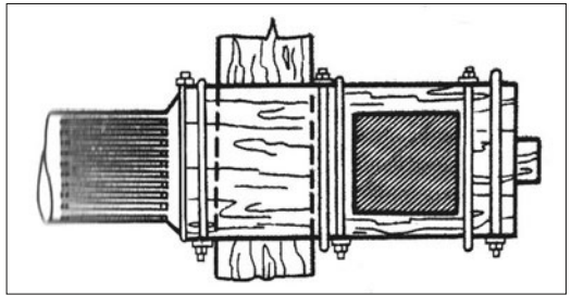
21 pav. Sparninio veleno medinis kaklas ir galva
