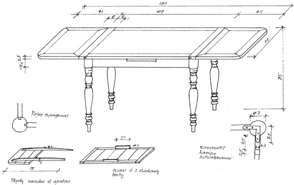
26 pav. Stalas. Kirmiškų k. Braižė D. Sabaliauskienė
