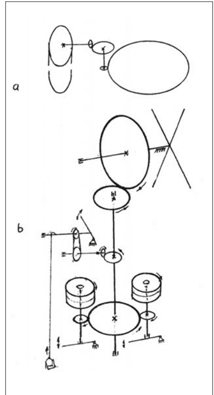
28 pav. Rogupių k. kepurinio vėjo malūno kinematinės schemos:
