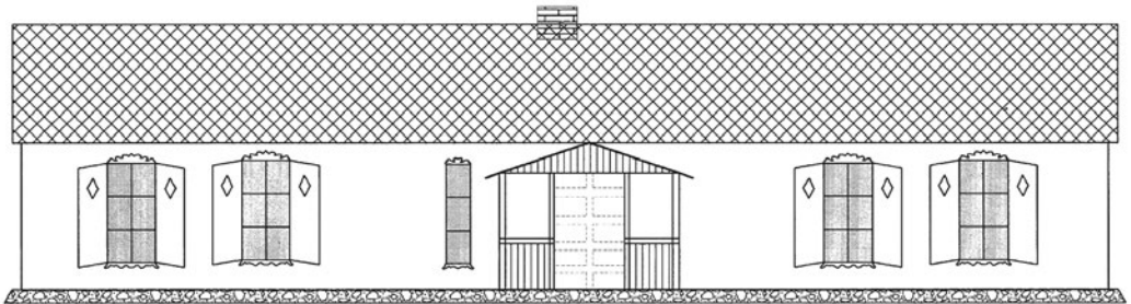
2 pav. Gyvenamojo namo ( stubos ) pagrindinis fasadas. Pagal autorės eskizą braižė A. Dubikaltienė
