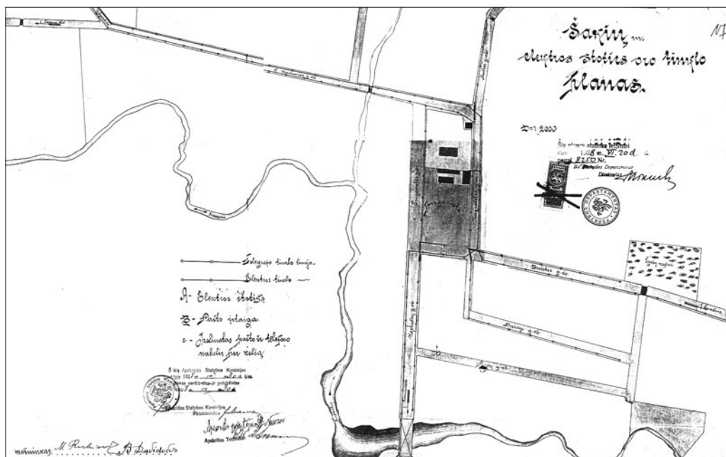
52 pav. Šakių elektros stoties oro tinklo planas
