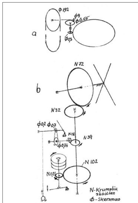
24 pav. Keturnauijenos k. kepurinio vėjo malūno kinematinės schemas:
