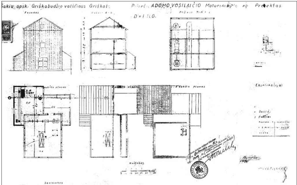
57 pav. Adomo Vosilaičio motorinio malūno projektas
