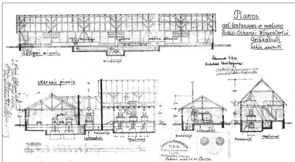
55 pav. Oskaro Vingendorfo lentpjūvės ir malūno pjūviai
