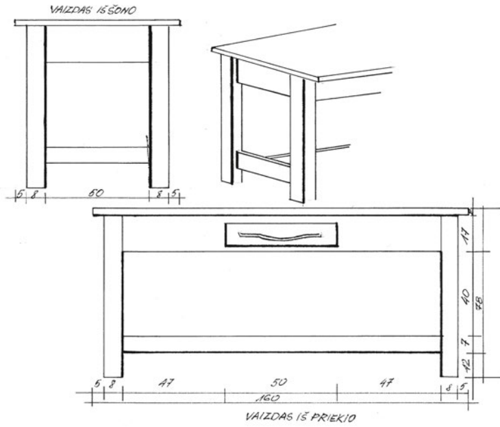
23 pav. Stalas. XIX a. vid. Sintautų mstl. Braižė Laura Bomblauskienė
