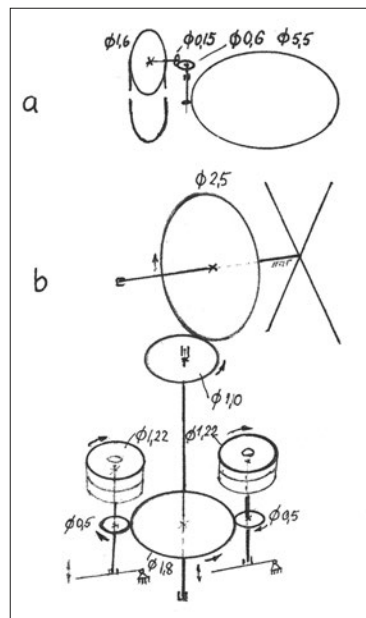
40 pav. Otto Kyno vėjo malūno Daugėliškio k. kinematinės schemos: a) kepurės apgręžimo krumpliaratine pavara kinematinė schema, b) malūno ir maišų užkėlimo mechanizmo kinematinė schema
