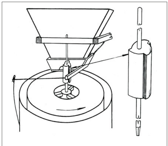
19 pav. Stiebinio malūno grūdų įberimo mechanizmas
