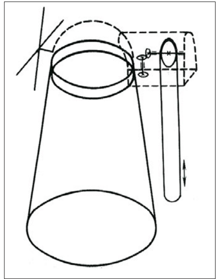
11 pav. Kepurės apgrėžimo krumpliartine pavara kinematinė schema
