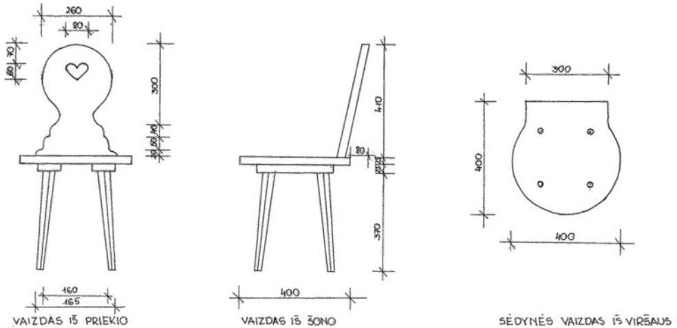
31 pav. Suolelis. Sintautų mstl. Braižė S. Stadalninkaitė
