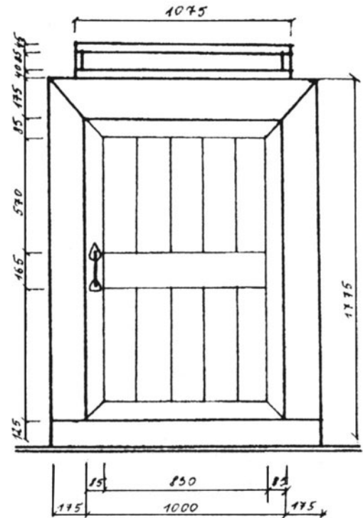
5 pav. Lauko durys (mm)
