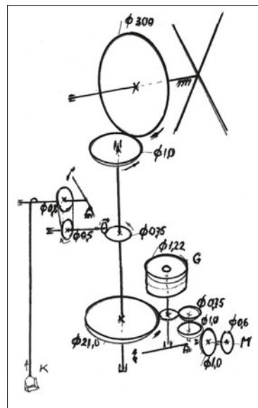
71 pav. A. Vosylaičio vėjo malūno kinematinė schema
