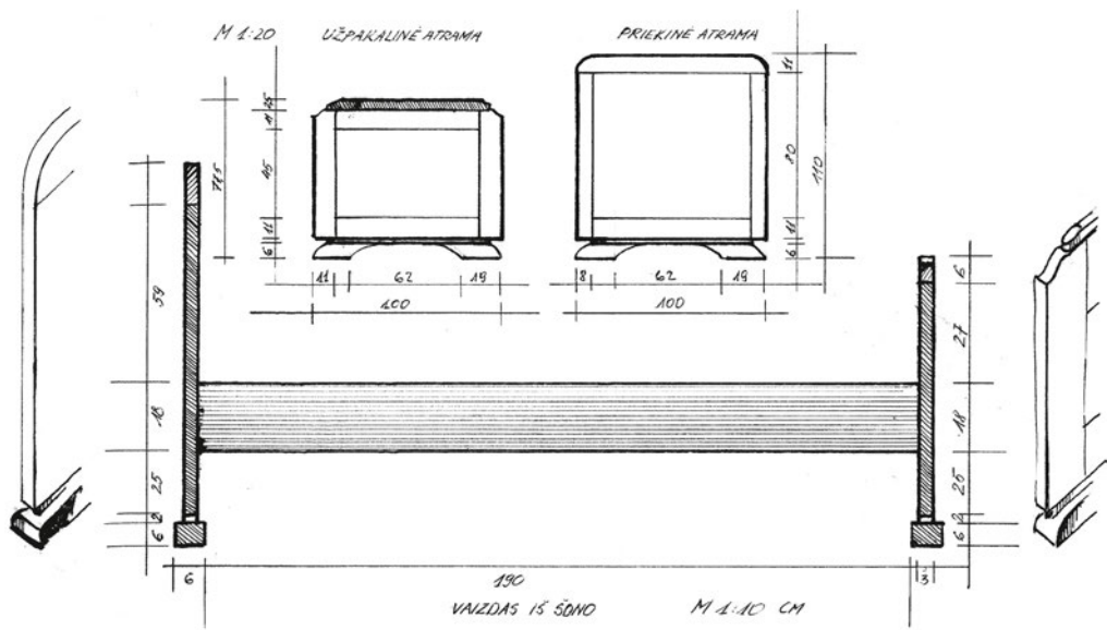
39 pav. Lova. XX a. 4-as dešimtmetis. Sintautų mstl. Braižė L. Bomblauskienė
