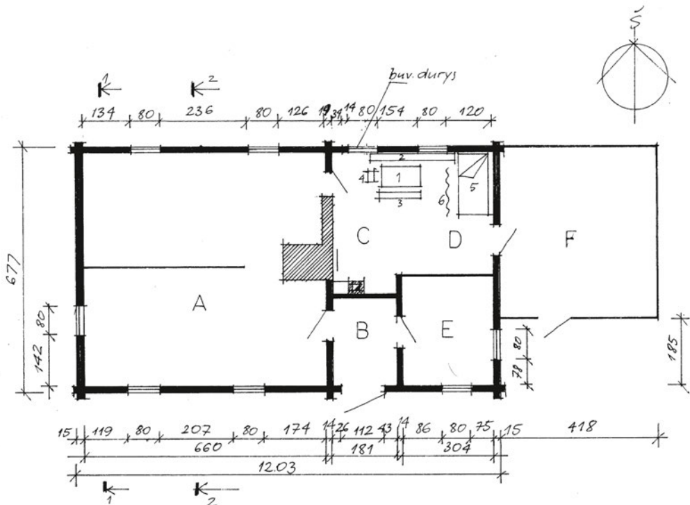
1 pav. Gyvenamojo namo, statyto XIX a. 2-ojoje pusėje, planas. Gaisrių k. Braižė Dovilė Sabaliauskienė
