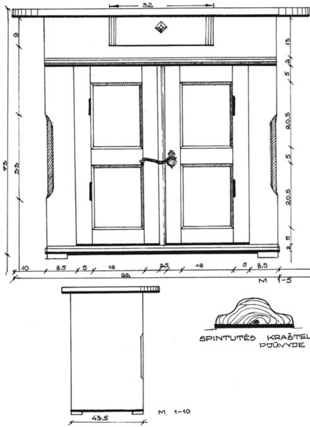
47 pav. Stalo tipo spintelė. Sintautų mstl. Braižė G. Stulgaitytė
