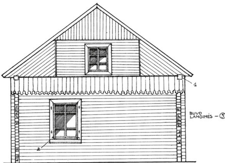
6 pav. Gyvenamojo namo, statyto 1915 m., fasadas. Gaisrių k. Braižė Daiva Šulgaitė
