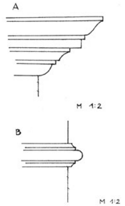
42 pav. Spinta. XIX a. 2-oji pusė. Sintautų mstl. Braižė D. Šulgaitė
