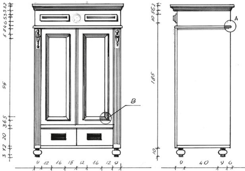
44 pav. Spinta. XX a. pr. Voverių k. Braižė L. Aleksandravičius
