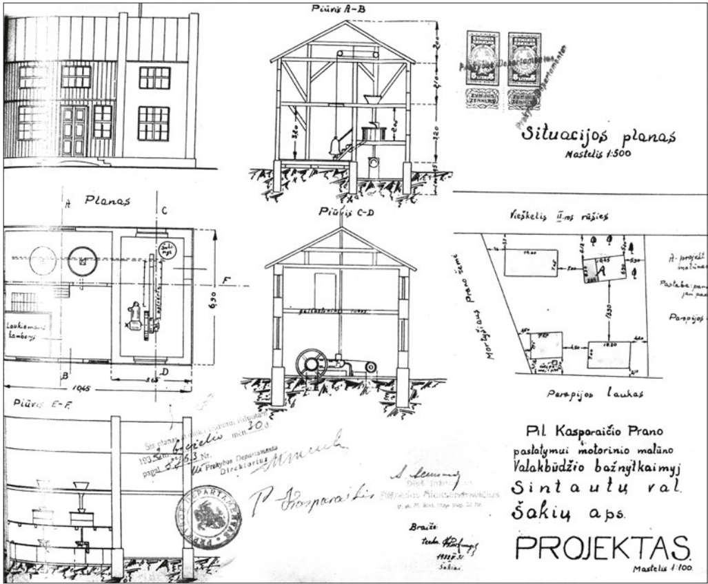
62 pav. P. Kasperaičio motorinio malūno projektas
