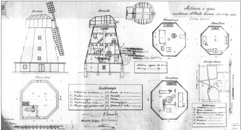
60 pav. A. Ešiaus vėjo-motorinis malūnas
