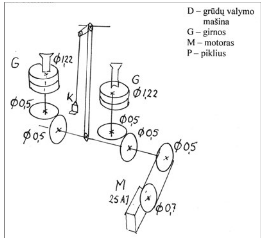
63 pav. P. Kasperaičio malūno kinematinė schema
