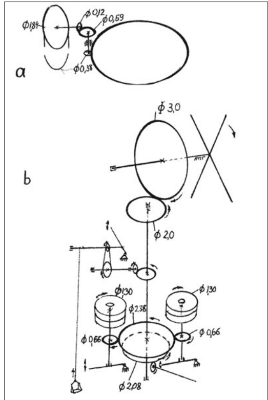
5 pav. Alg. Maksvyčio kepurinio malūno kinematinės schemas: a) kepurės apgręžimo krumpliaratine pavara kinematinė schema, b) malūno ir mairių užkėlimo mechanizmo kinematinė schema
