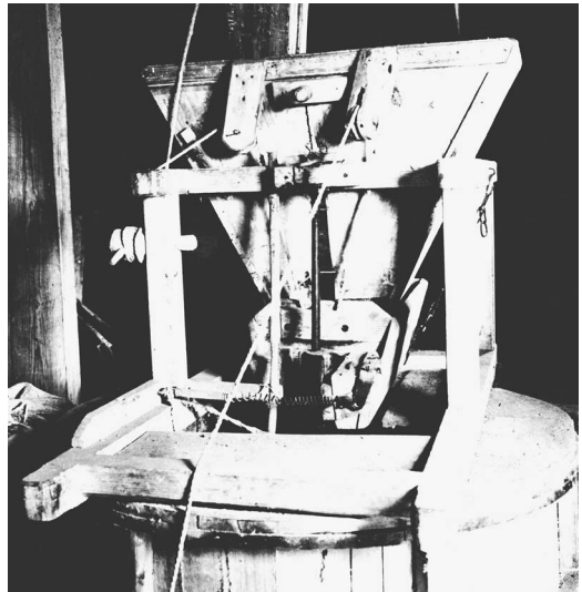
6 pav. Grūdų įbėrimo mechanizmas statomas ant girnų kubilo
