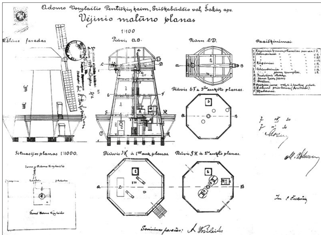
70 pav. A. Vosylaičio vėjo malūno planas
