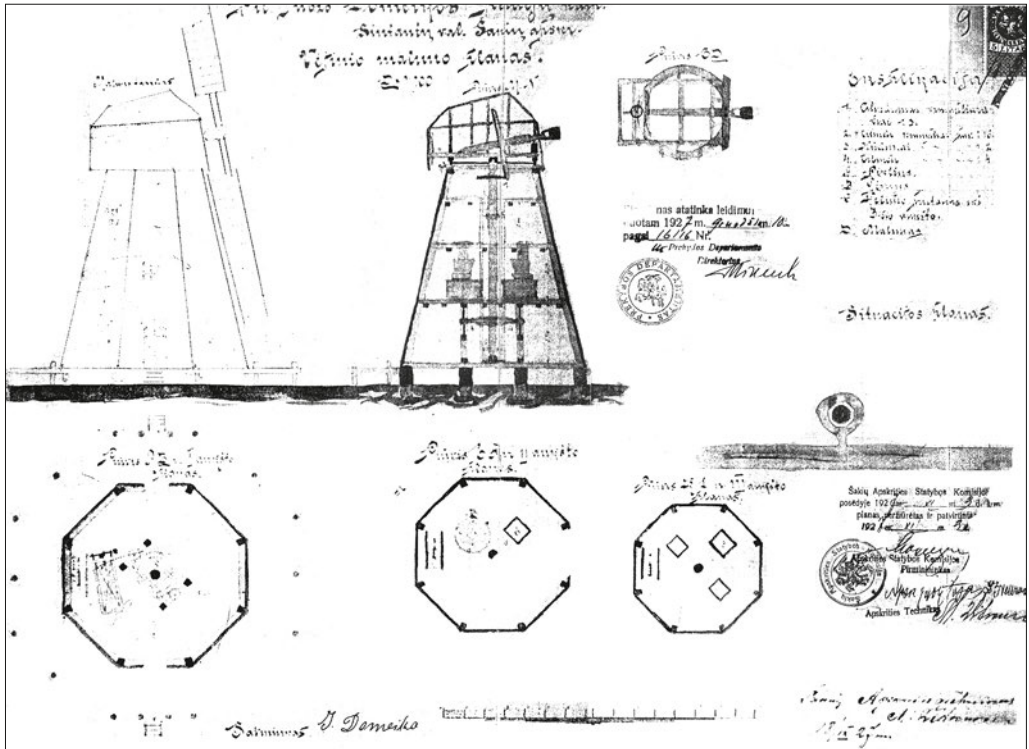
29 pav. Juozo Domeikos Išdagų k. kepurinio malūno planas
