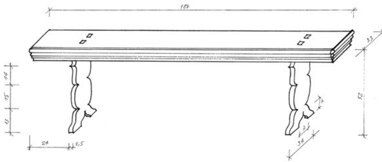
28 pav. Suolas. Kirmiškių k. Braižė D. Sabaliauskienė
