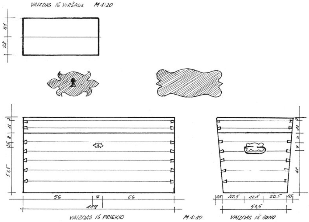
40 pav. Skrynia. 1820 m. Sintautų mstl. Braižė L. Bomblauskienė
