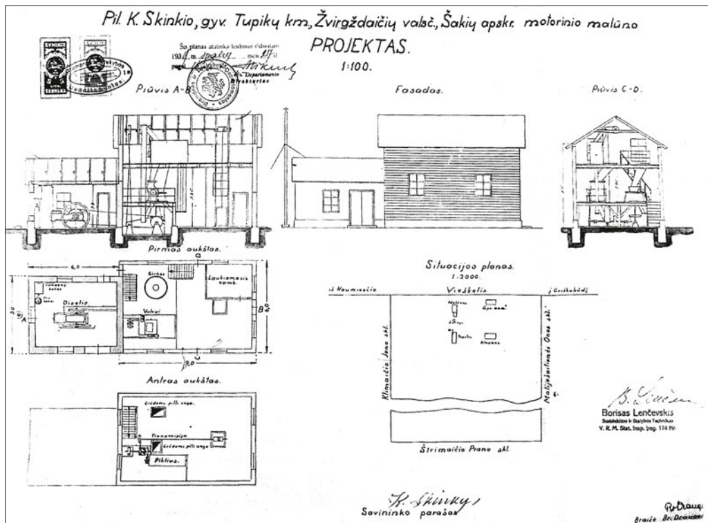
66 pav. K. Skinkio motorinio malūno projektas
