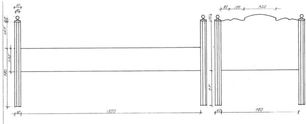
38 pav. Lova. 1930 m. Urbantų k. 1930 m. Braižė Daiva Domereckaitė
