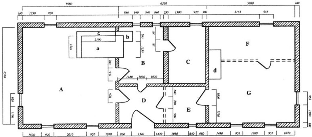
1 pav. Gyvenamojo namo (stubos) planas (mm). A – stuba, B – virtuvė, C – grinčiūtė, D – priemenė, E – priestubys, F – stubeliukė, G – stubelė; a – krosnis, b – viryklė, c – zelikis, d – pečiukas (statukas)
