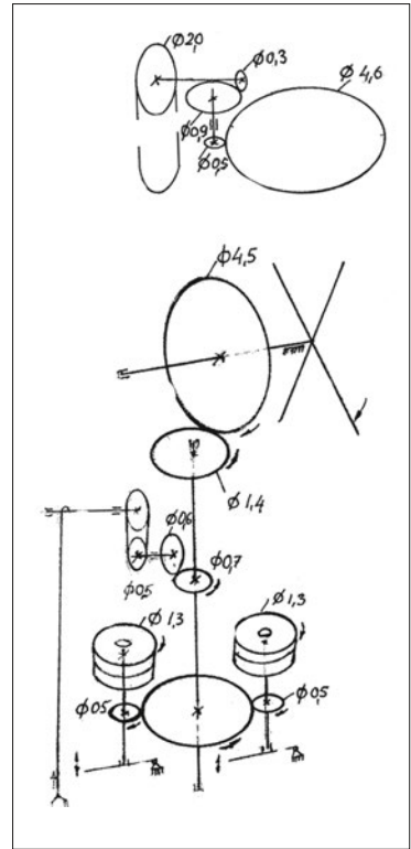
49 pav. Antaninos Spurgienės vėjo malūno Šunkarių kaime kinematinės schemas
