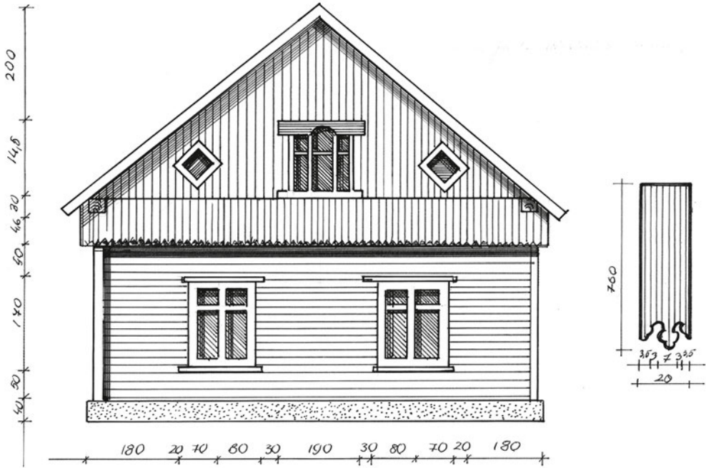
RYTINIS FASADAS M : 1:50
