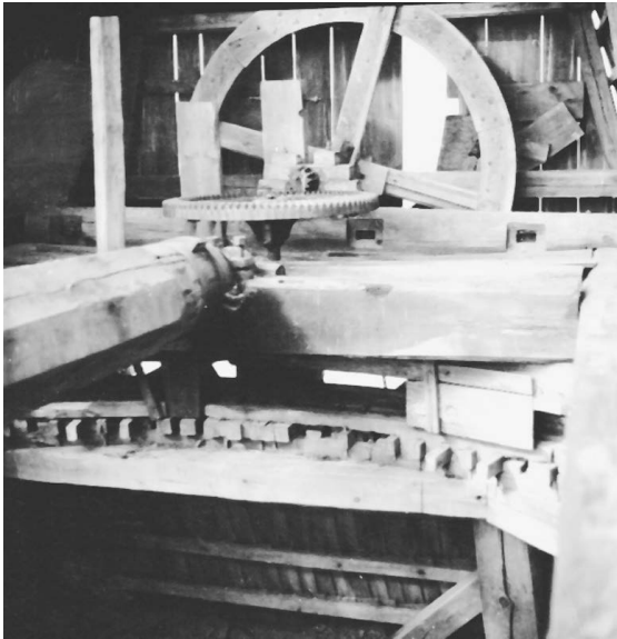
10 pav. Kepurės apgrėžimas krumpliartine pavara
