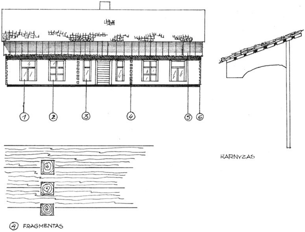
11 pav. Gyvenamojo namo fasadas. Sintautų mstl. Braižė Vilija Mostauskytė
