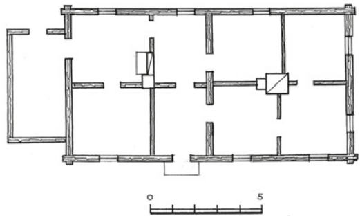
14 pav. Vytautavos klebonijos planas. Sudarė A. Rupeika
