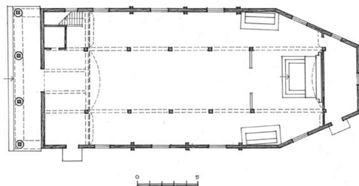
10 a pav. Dusmenų bažnyčios planas. Sudarė A. Rupeika
