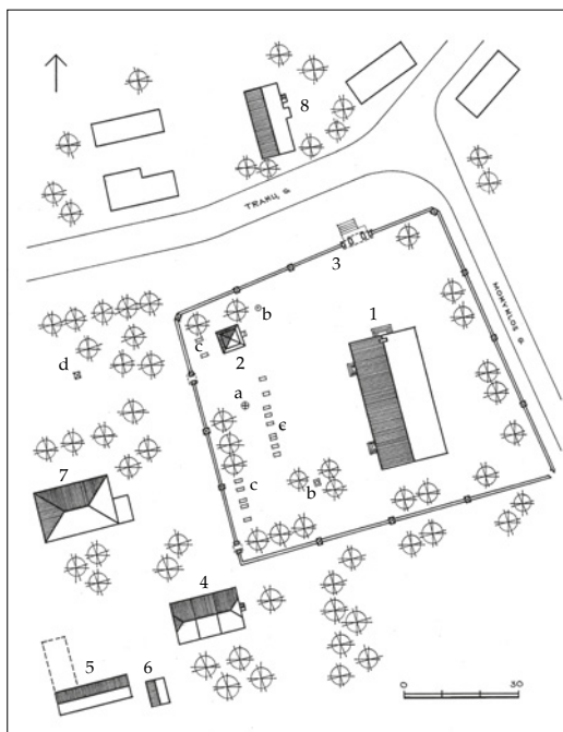
3 pav. Onuškio bažnyčios statinių ir klebonijos trobesių situacijos plano schema. 1) bažnyčia; 2) varpinė; 3) šventoriaus tvora su vartais ir Kryžiaus kelio stočių koplytėlėmis, a) kryžius, b) paminklas, c) kapas, d) stogastulpis; 4) klebonija; 5) ūkinis trobesys; 6) ūkinis trobesys; 7) parapijos pastatas; 8) špitolė.
