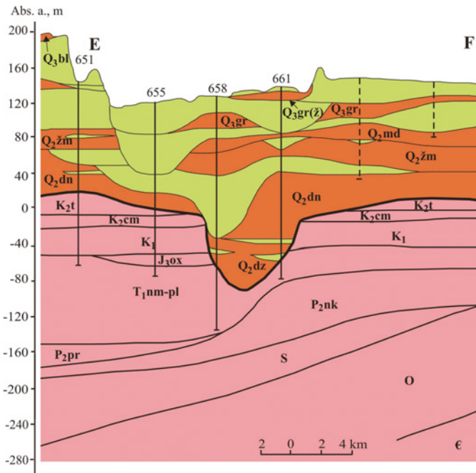
4 pav. Geologinis pjūvis E–F. Sutartiniai ženklai prie 2 pav. Sudarė A. Šliaupa, V. Baltrūnas, B. Karmaza
