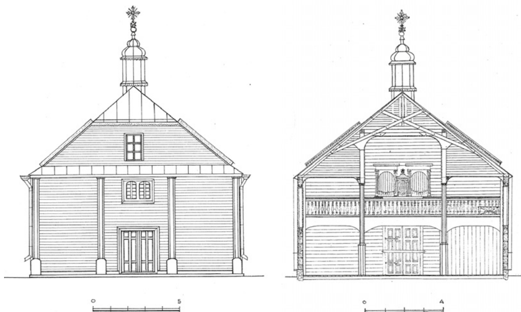
10 b pav. Dusmenų bažnyčios pagrindinis fasadas. ASI
