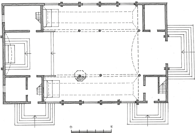
16 pav. Žilinių bažnyčios planas. Sudarė A. Rupeika
