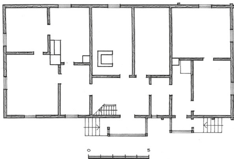
7 pav. Onuškio špitolės planas. Sudarė A. Rupeika
