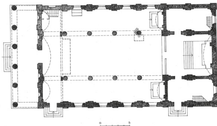
4 a pav. Onuškio bažnyčios planas. Sudarė A. Rupeika
