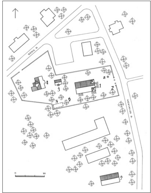
15 pav. Žilinių bažnyčios statinių ir klebonijos trobesių situacijos plano schema. 1) bažnyčia; 2) šventoriaus tvora su vartais, a) kryžius; 3) laikinoji klebonija; 4) klebonija; 5) ūkinio trobesio vieta; 6) šulinys; 7) špitalė (senoji klebonija). Sudarė A. Rupeika
