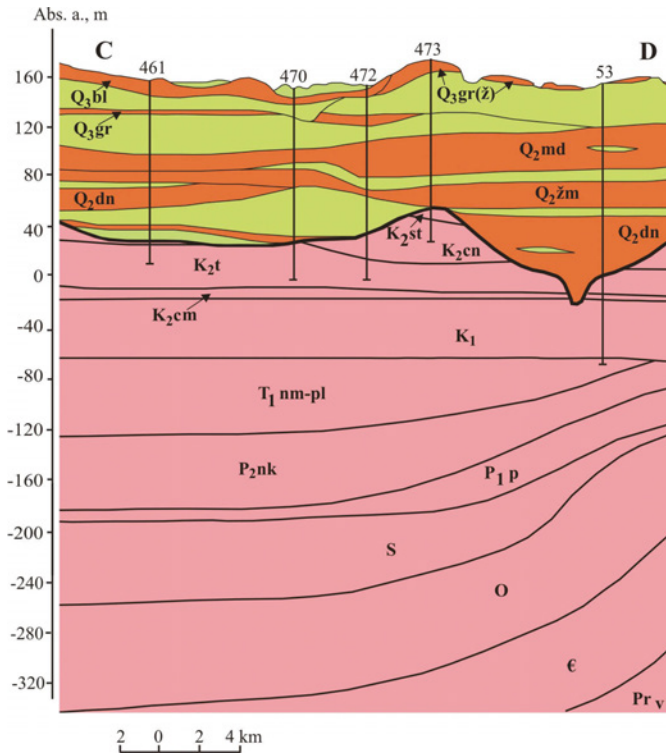
3 pav. Geologinis pjūvis C–D. Sutartiniai ženklai prie 2 pav. Sudarė A. Šliaupa, V. Baltrūnas, B. Karmaza
