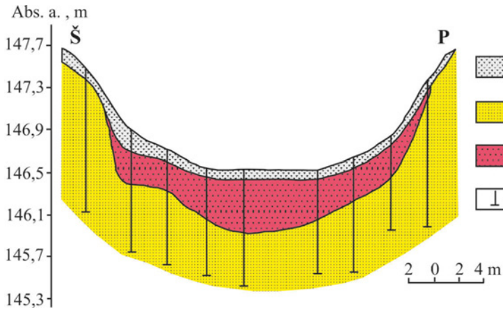
10 pav. Lobo su raudonžemiu geologinis pjūvis. 1 – dirvožemis; 2 – smulkus šviesiai geltonas smėlis; 3 – smulkus ir smulkutis raudonasis smėlis; 4 – grėžinys
