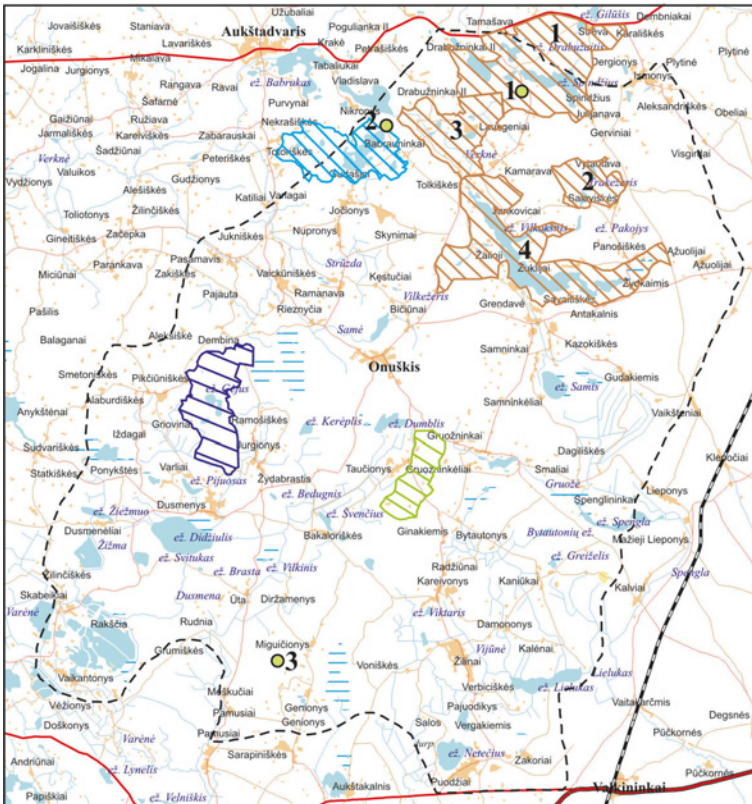
4 pav. Žemiau tįsančios Baltijos stadijos smulkios kalvos prie Taučionių
