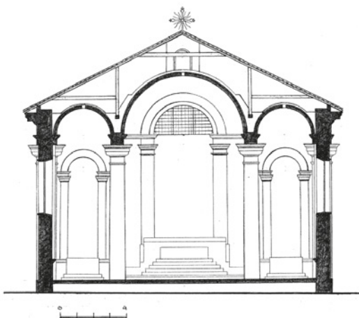
4 c pav. Onušio bažnyčios skersinis pjūvis. ASI
