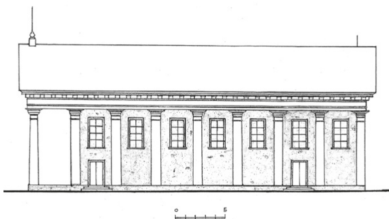
4 b pav. Onuškio bažnyčios vakarų fasadas. ASI
