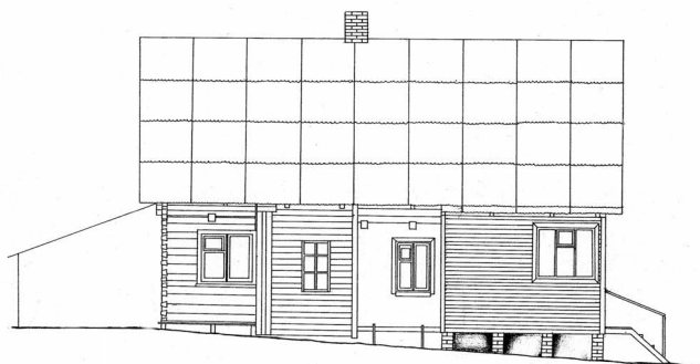
ŠIAURĖS VAKARŲ FASADAS M 1:50
