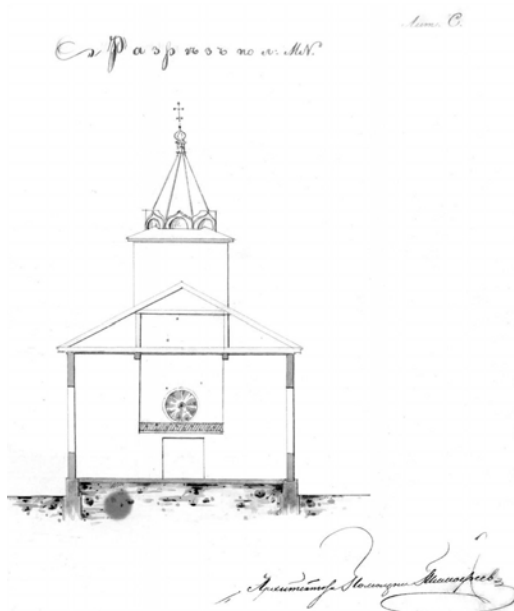
1848 m. medinės bažnyčios projektas (neįgyvendintas), autorius – architekto padėjėjas M. Timofejevas. Viršuje – fasadas AB, apačioje – pjūvis MN
