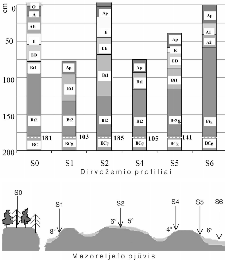
1 pav. Mezoreljefo fragmentas ir dirvožemio nuardymo laipsnis Laukuvos seniūnijos Mažųjų Vankių kaime. S0–S6 – dirvožemio profiliai: S0 – sąlyginai nenuardytas dirvožemis miške; S2 – menkai nuardytas dirvožemis; S5 – vidutiniškai nuardytas; S1 ir S4 – labai nuardytas; S6 – užneštas dirvožemis. Dirvožemių profilių vietos nurodytos rodyklėmis. Balta punktyrinė linija rodo karbonatingojo horizonto gylį cm
