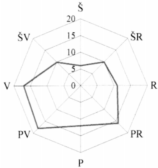
Laukuvos MS daugiametė vėjų rozė
