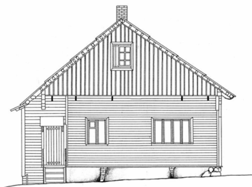
PIETVAKARIŲ FASADAS M 1:50
