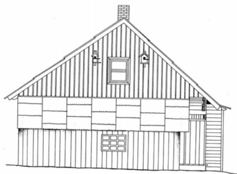
ŠIAURĖS RYTŲ FASADAS M 1:50
