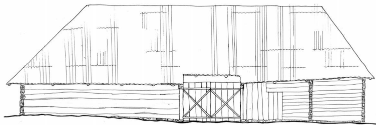
46 pav. Sodybos Nr. 28 tvarto stogo konstrukcijos fragmentas. 2001 m.
