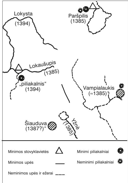
Kryžiuočių karo kelių aprašymuose minimi Laukuvos apylinkių vietovardžiai. V. Almonaičio schema, 2002 m.
