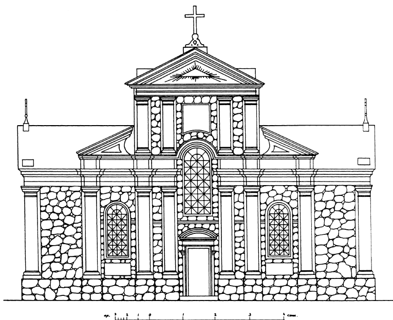
7 pav. Gelvonų bažnyčios pagrindinis fasadas. 1895 m. Sudarė architektas A. Polozovas. GBA
