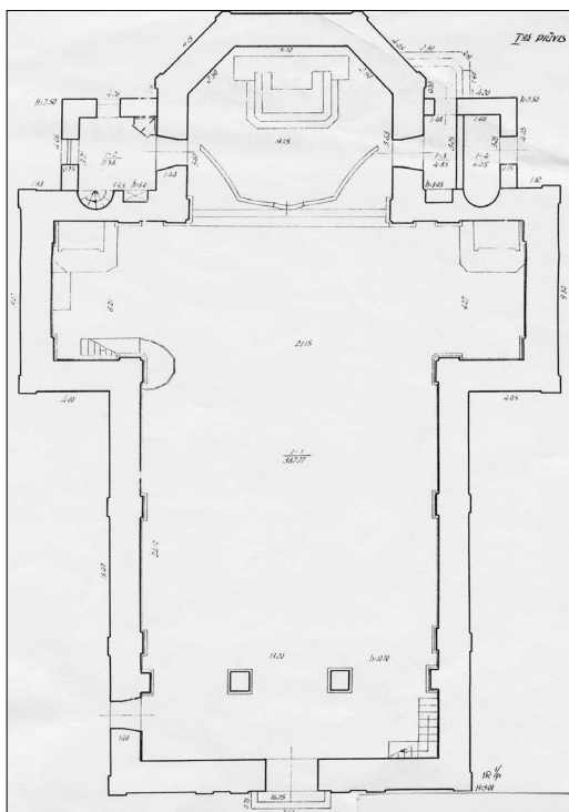
Gelvonų bažnyčios planas. M 1:100 1961 m. Braižė E. Gudonienė
