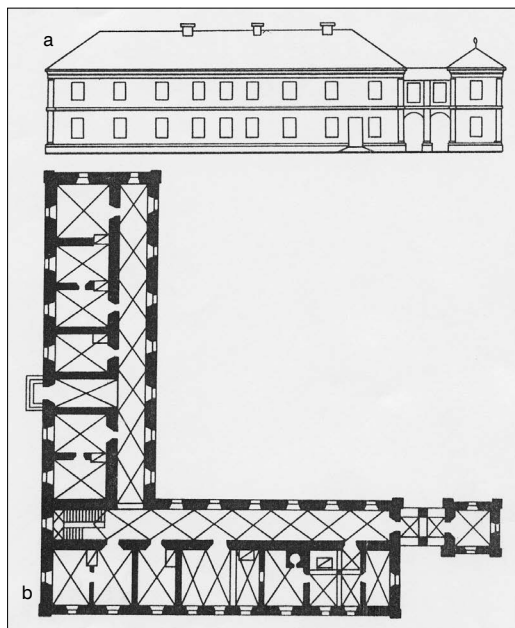
Gelvonų pranciškonų vienuolyno rekonstrukcija: a – fasadas, b – pirmojo aukšto planas. Iš kn. „Lietuvos architektūros istorija“, Vilnius, 1992, t. 2, p. 291
