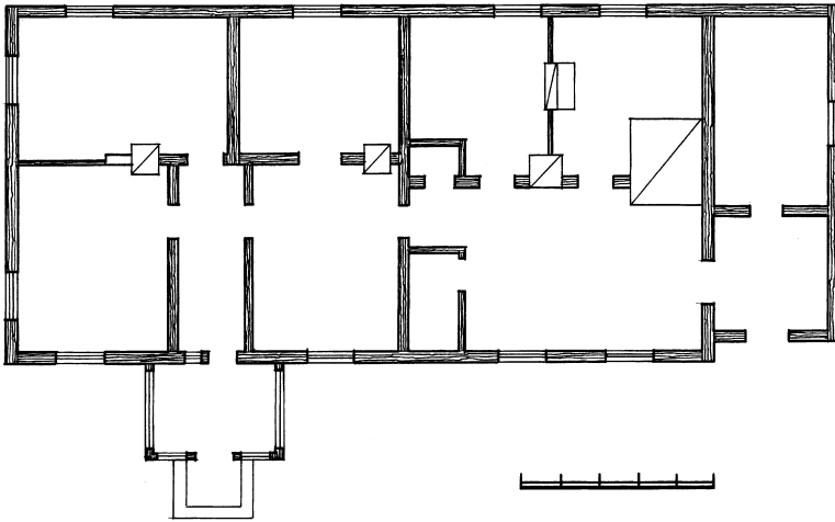
28 pav. Boleslavos dvaro namo planas
