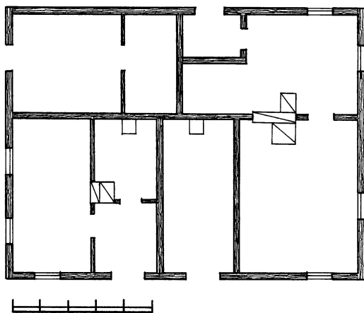
20 pav. Namas Mikalajūnų g. 6 planas. 2004 m. Braižė A. Rupeika
