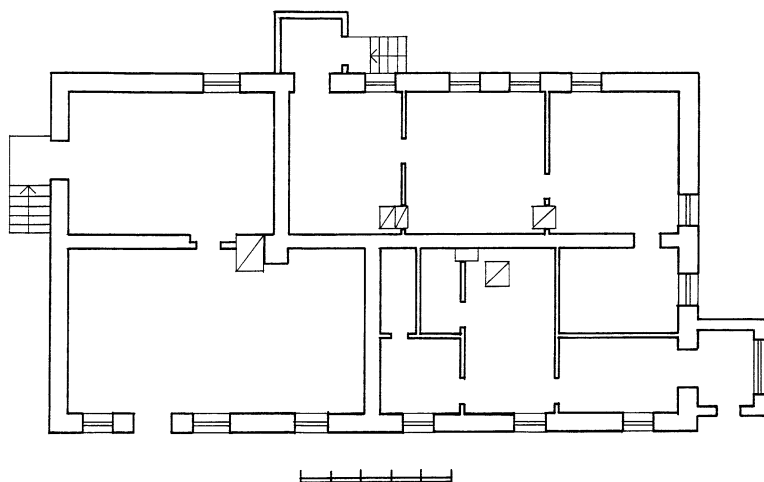
19 pav. Pastato Mikalajūnų g. 3 planas. 2004 m. Braižė A. Rupeika
