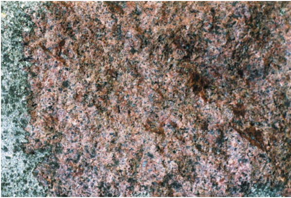
49 pav. Alandų rapakivis. 48 statinys. 161 blokelis. Regimas plotis – 39 cm. Kairiajame pakraštyje – cementas
