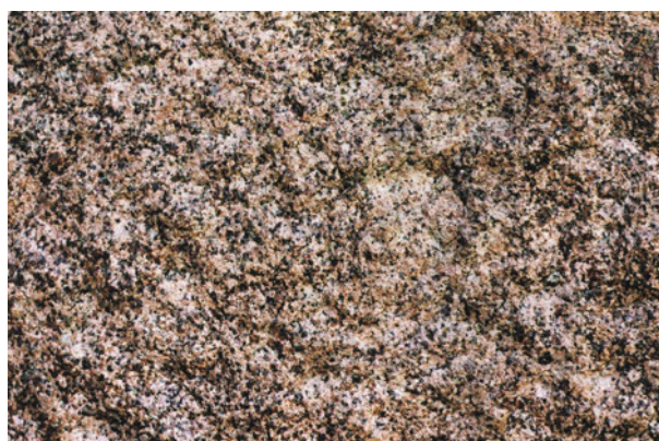
41 pav. Alandų granitas – rapakivis (Eckero tipo). 5 statinys. 15 blokelis. Matomas plotis – 35 cm
