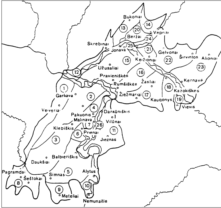
1 pav. Nemuno vidurupio ir Neries žemupio plynaukštės mikrorajonai
