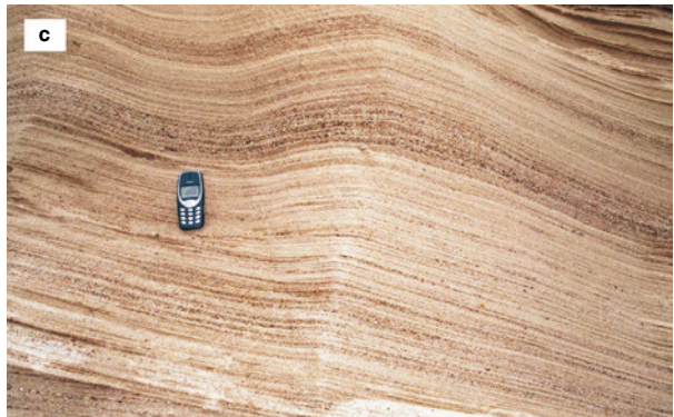
7 pav. Kraštinio fluvio-glacialinio gūbrio sandara Šiaulių telkinio Sedūnų karjere ryčiau Bagaslaviškio:
