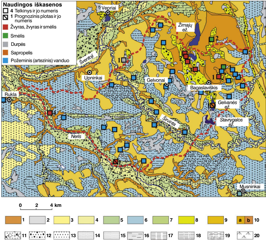
3 pav. Gelvonų apylinkių geologinis ir naudingųjų iškasenų žemėlapis.
