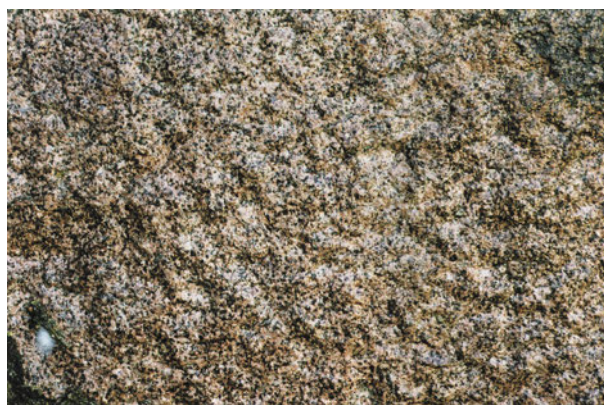
43 pav. Upsalos granitas. 4 statinys. 12 blokelis. Matomas plotis – 13 cm. Viršuje – cementas
