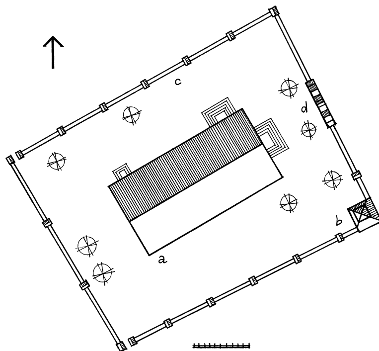
3 pav. Bagaslaviškio sakralinių statinių komplekso situacijos planas:
