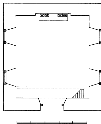
7 pav. Pyplių kapinių koplyčios planas. Apmatavimo brėžinys
