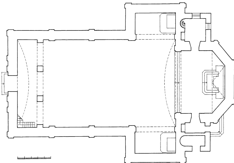
6 pav. Bažnyčios planas. 2004 m. Sudarė A. Rupeika
