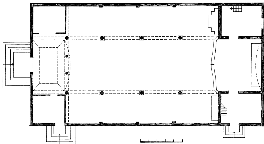
4 pav. Bagaslaviškio bažnyčios planas
