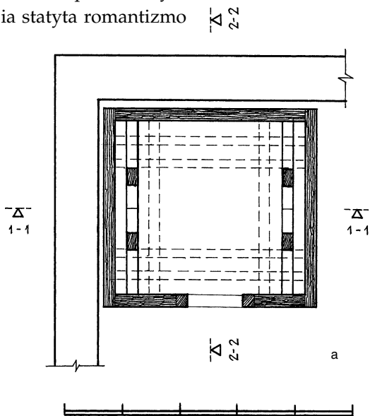
5 pav. Bagaslaviškio varpinės planas: a – apmatavimo brėžinys; b – pjūvis 1:1; c – pjūvis 2:2
