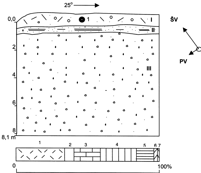
5 pav. Bagdyšių karjero prakasos pjuvis, gargždo petrografinės sudėties integralinė diagrama ir orientacijos maksimumų krypčių strėlės:
