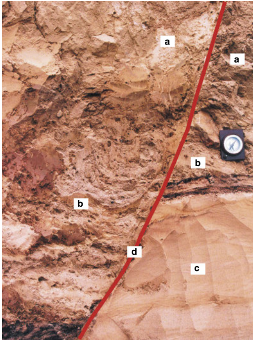
8 pav. Ledyno dislokuoti sluoksniai moreniniame masyve Jutkonių karjere į šiaurę nuo Gelvonų: a – moreninis priemolis; b – sujauktas smėlis ir molis su retu gargždu; c – smulkus ir gerai išrūšiuotas smėlis; d – sprūdžio linija. 2003 m.
