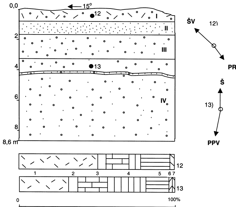
4 pav. Zubelių karjero prakasos pjūvis, gargždo petrografinės sudėties integralinės diagramos ir orientacijos maksimumų krypčių strėlės:
