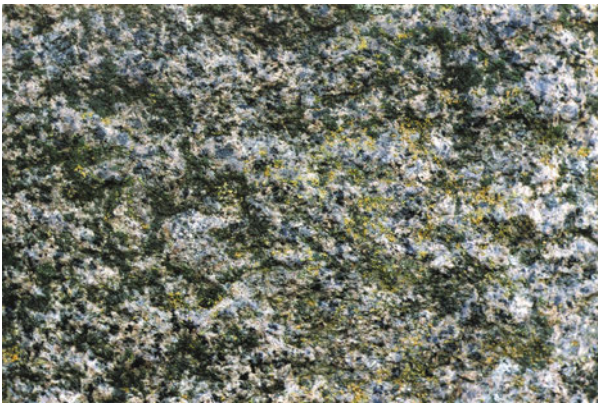
52 pav. Alandų granitas. 48 statinys. 162 blokelis. Matomas plotis – 20 cm. Viršuje matyti cementas
