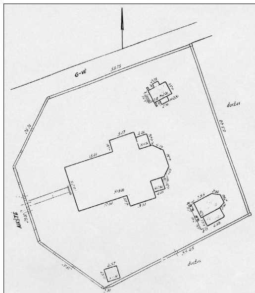
Gelvonų bažnyčios šventoriaus ir ansamblio planas. 1961 m. Braižė E. Gudonienė
