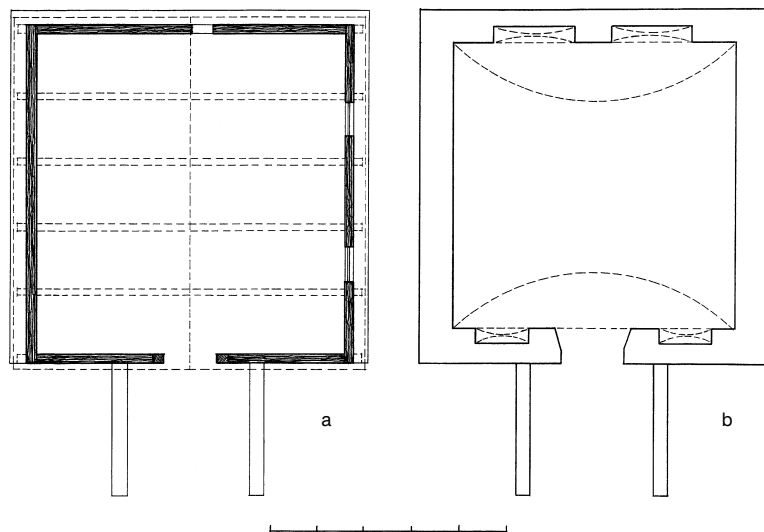
19 pav. Gelvonų dvaro svirnelio-ledainės apmatavimo brėžiniai: a – I a. planas; b – rūsio planas
