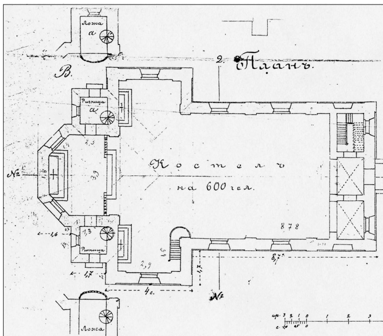
Gelvonų bažnyčios planas. Architektas A. Polozovas. 1895 m. GBA
