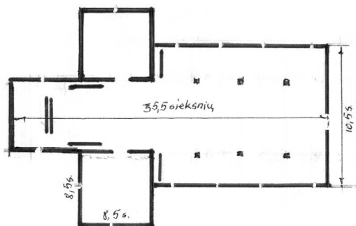
Barokinės bažnyčios plano schema pagal 1820 m. vizitaciją. 2007 m. Braižė P. Spurgevičius
