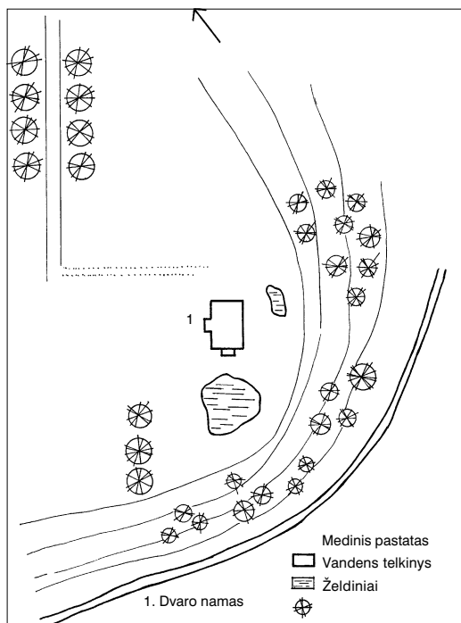
26 pav. Šiaulių dvaro sodybos situacijos schema
