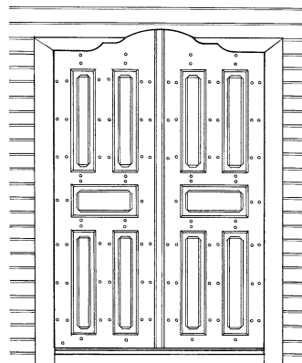
18 pav. Gelvonų Kapinių koplyčios durų apmatauimo brėžinys. 2004 m.
