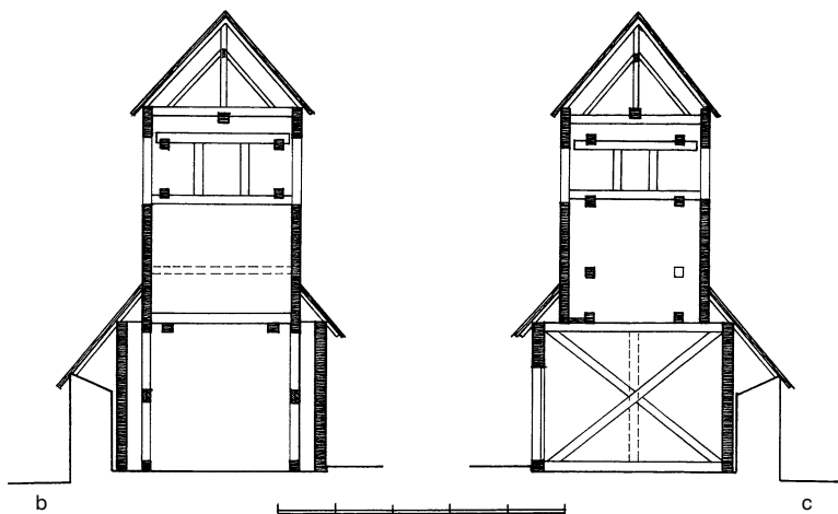
6 pav. Bagaslaviškio varpinės pjūvis: pjūvis 1:1 (b); pjūvis 2:2 (c)
