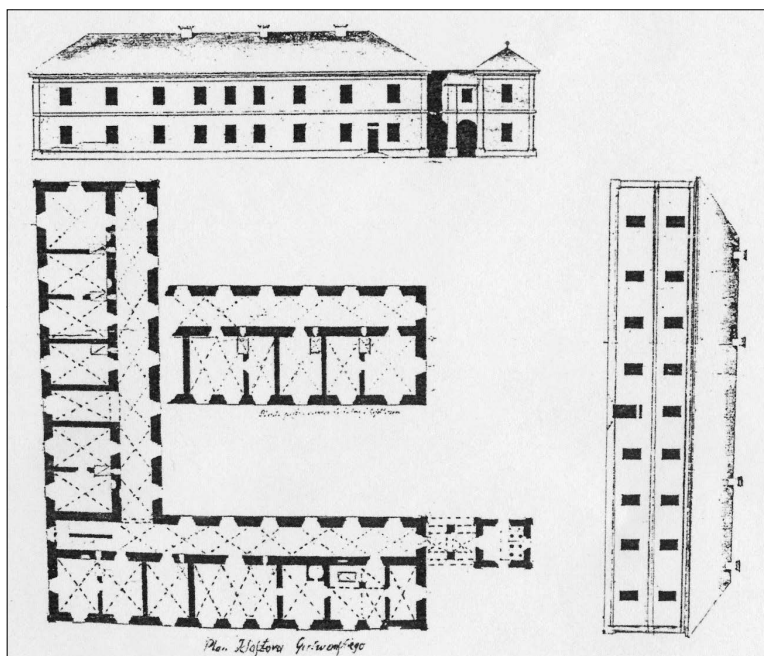
Gelvonų vienuolyno planas ir fasadas. Archit. K. Kaminskis. 1788 m.
